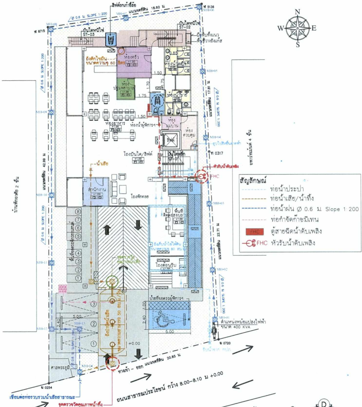
รูปที่ 5 : แผนผังจุดตรวจวัดคุณภาพสิ่งแวดล้อมช่วงดำเนินการ
