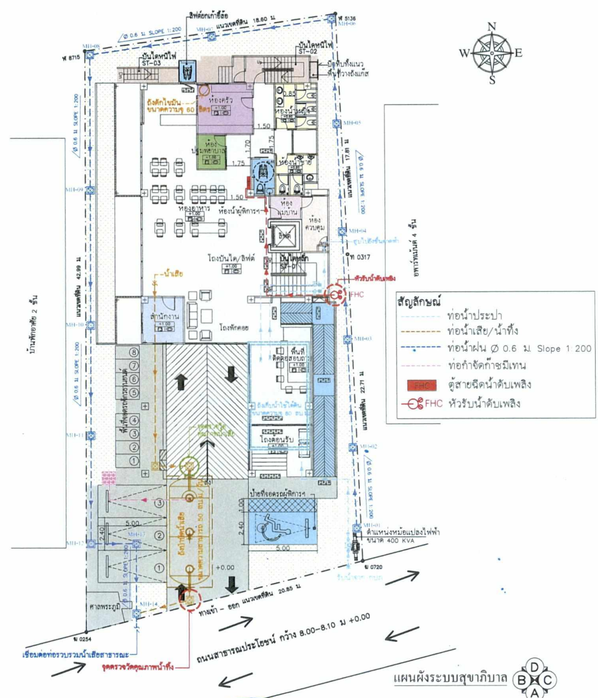
รูปที่ 1 - แผนผังระบบสุขาภิบาล
