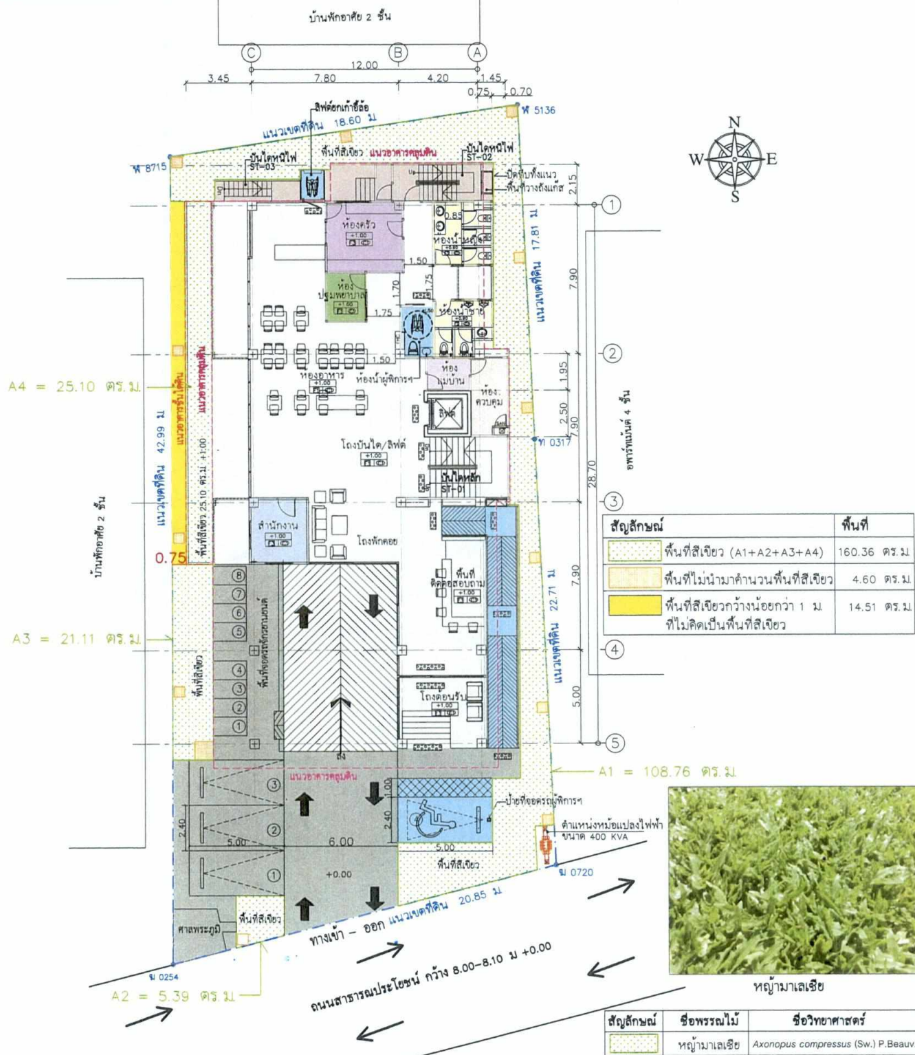
แผนผังพื้นที่สีเขียว
