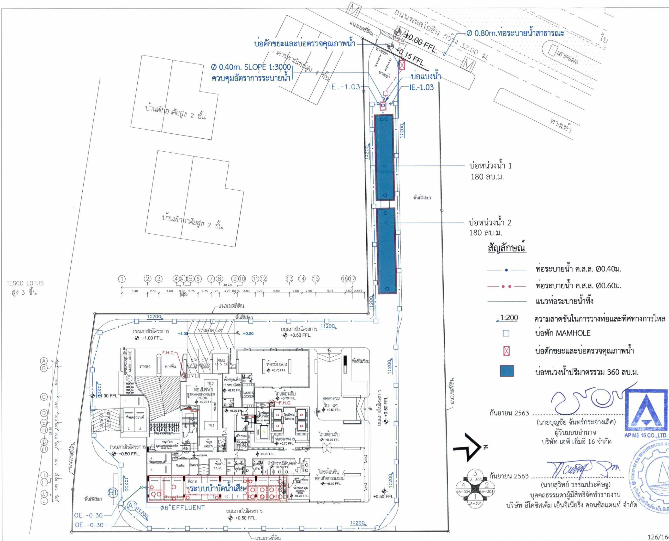
ภาพที่ 5 ผังระบบระบายน้ำและบ่อหน่วงน้ำ
