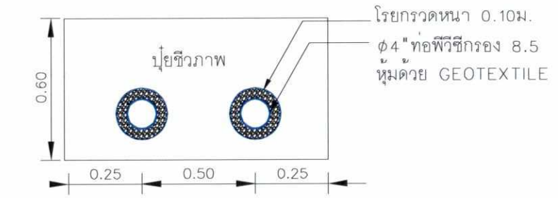
รูปแสดงพื้นที่หน้าตัดบ่อกำจัดมูลด้วยปุ๋ยชีวภาพ
