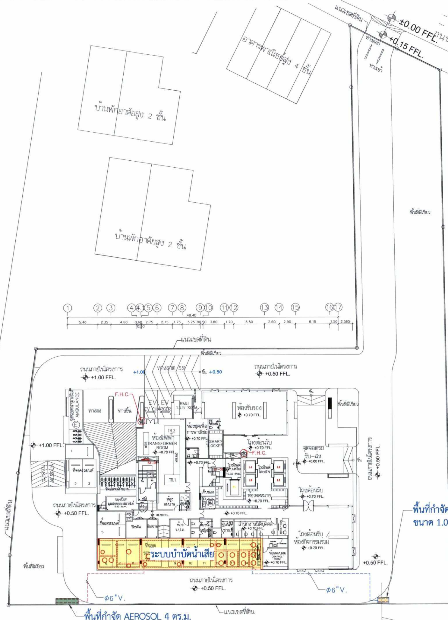
ภาพที่ 6 ผังระบบบำบัดน้ำเสีย
