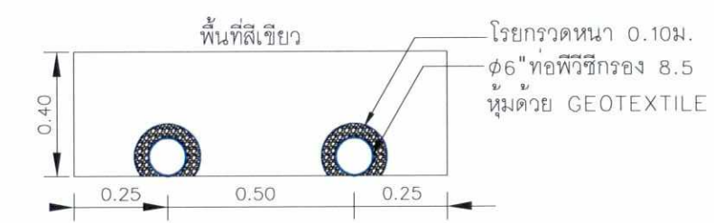
รูปแสดงพื้นที่หน้าตัดบ่อกำจัด AEROSOL
