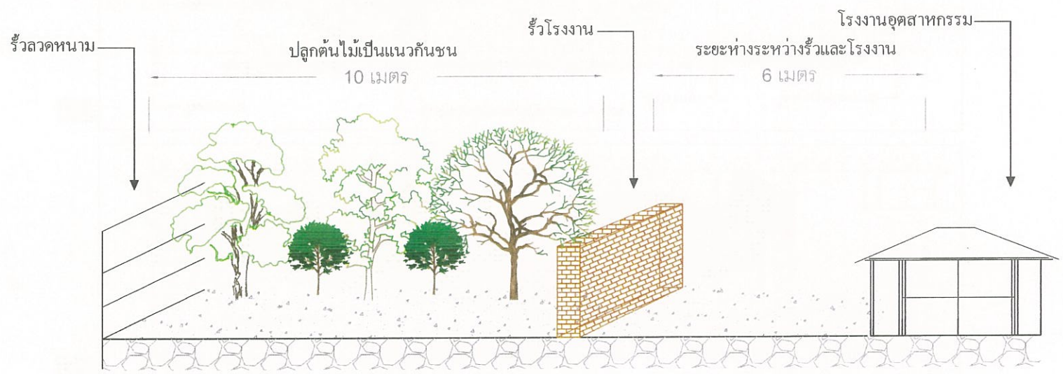
รูปที่ 5 ผังแสดงแนวกันชนบริเวณทางด้านทิศตะวันออกของโครงการ
