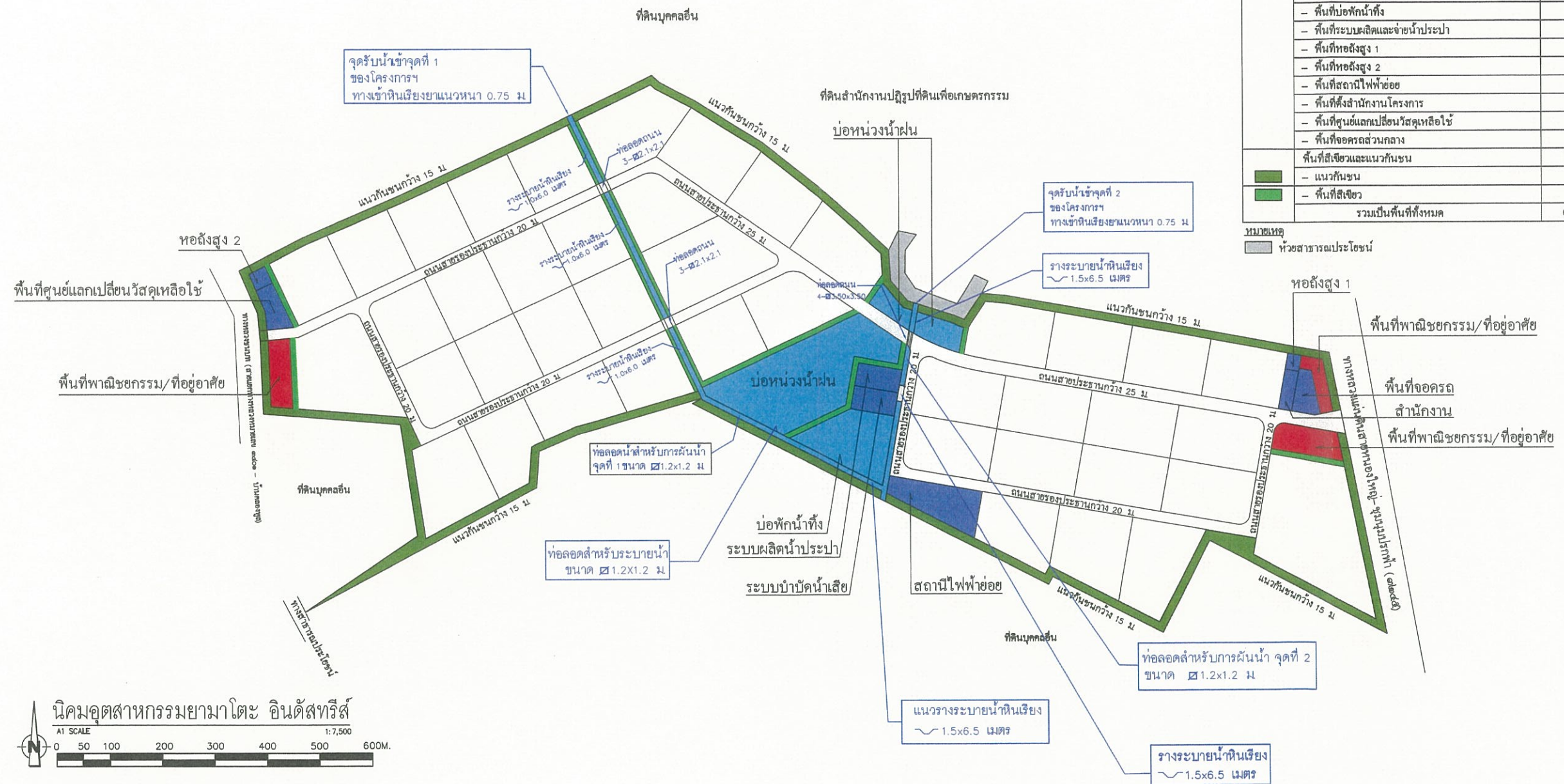
รูปที่ 7 ผังแสดงตำแหน่งจุดรับน้ำ
