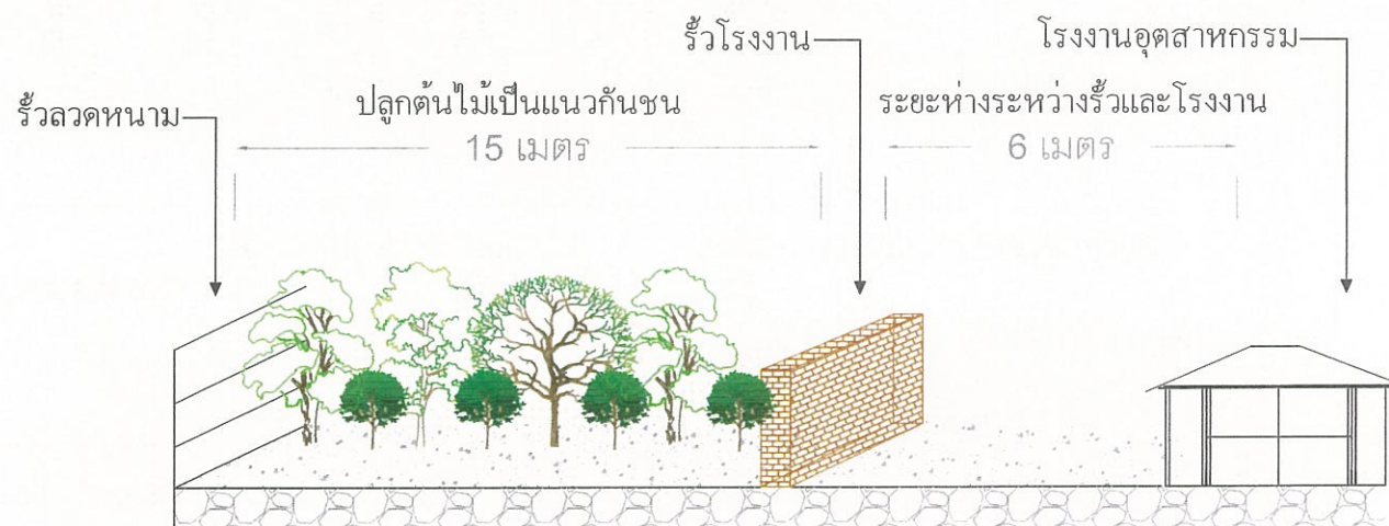
รูปที่ 3 ผังแสดงแนวกันชนบริเวณทางด้านทิศเหนือของโครงการ
