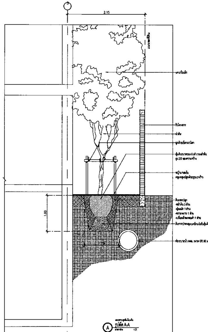
รูปที่ ผ.1-8 รูปตัด A-A การปลูกต้นไม้ภายในโครงการ
