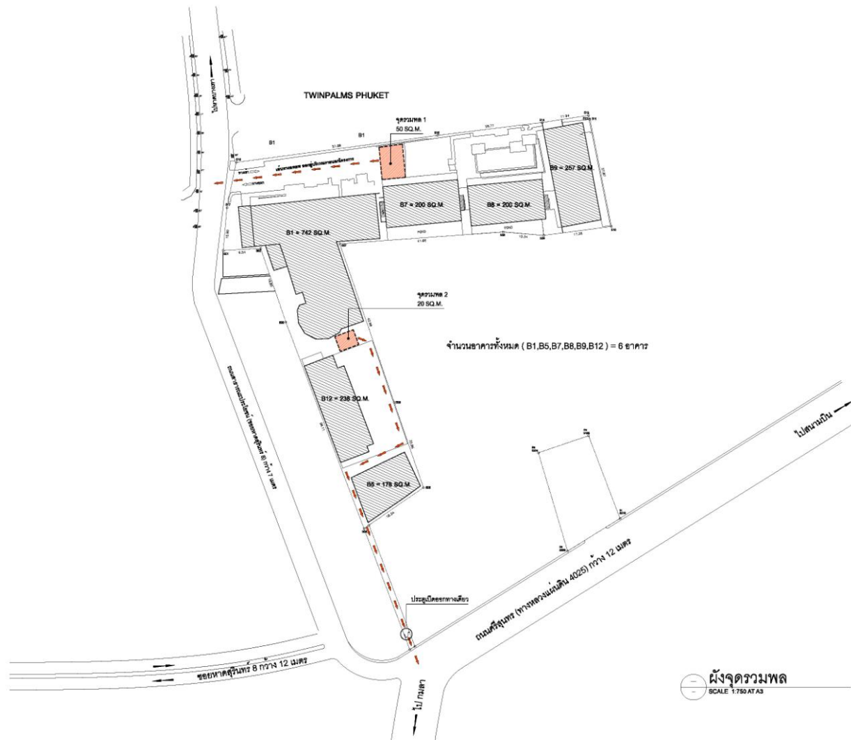
ภาพที่ 13 ผังบริเวณแสดงเส้นทางอพยพจากพื้นที่จุดรวมพล ออกสู่ภายนอกโครงการ
