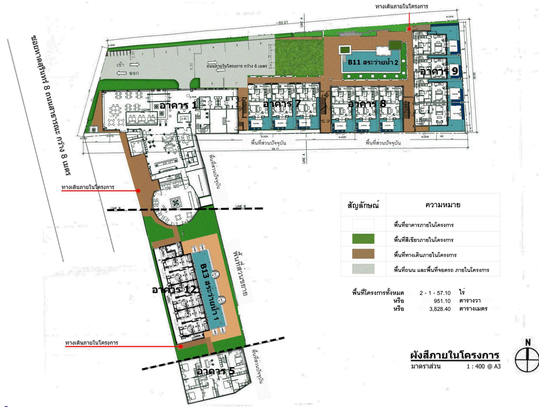
ภาพที่ 2 ผัง (สี) แสดงการใช้ประโยชน์พื้นที่โครงการ ภายหลังการก่อสร้างส่วนขยาย
