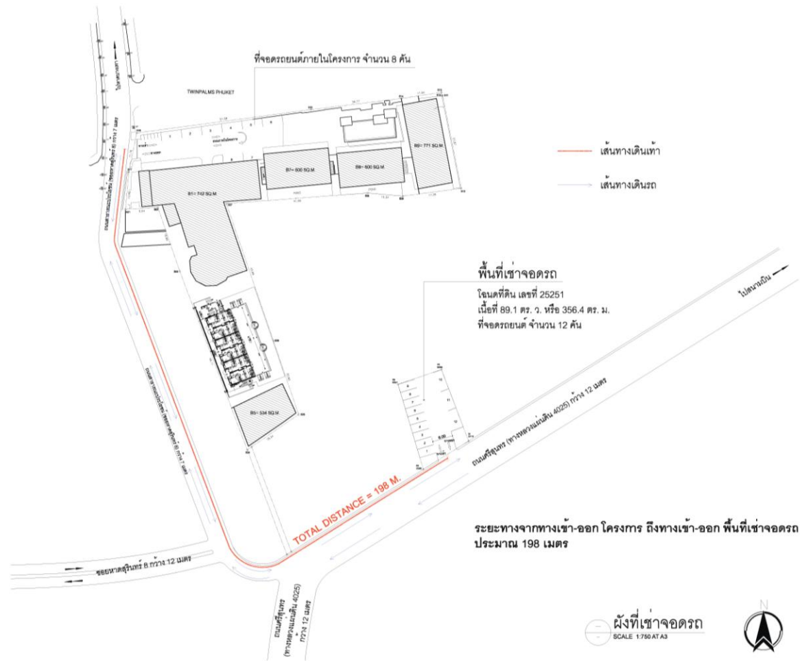
ภาพที่ 6 ผังบริเวณ แสดงทางเข้า-ออก ทิศทางการจราจรภายในโครงการ และที่จอดรถยนต์ 2 แห่ง
