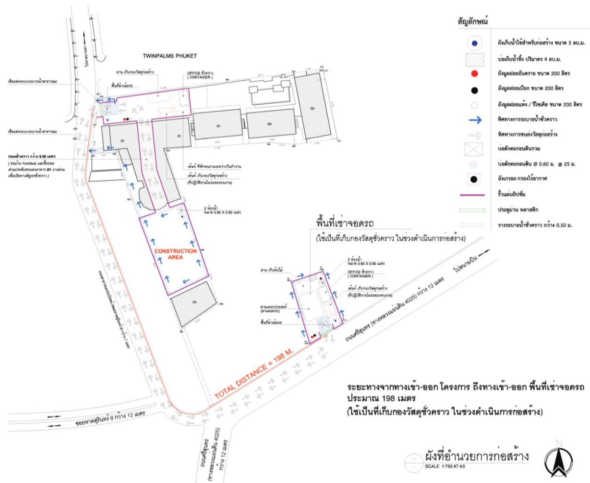
ภาพที่ 14 ผังบริเวณแสดงพื้นที่อำนวยความสะดวกก่อสร้าง และระบบสาธารณูปโภคในระหว่างการก่อสร้าง
