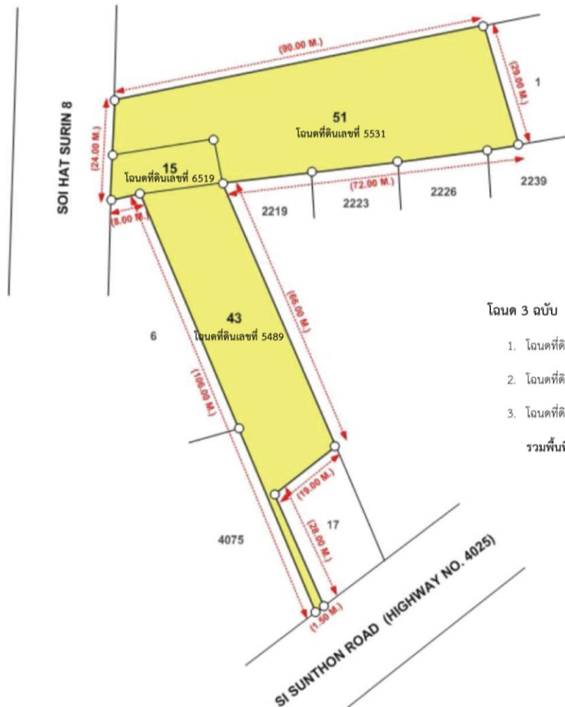
ภาพที่ 1 ผังต่อโฉนดที่ดินของโครงการ และถนนสาธารณะประโยชน์ (ซอยหาดสุรินทร์ 8 )
