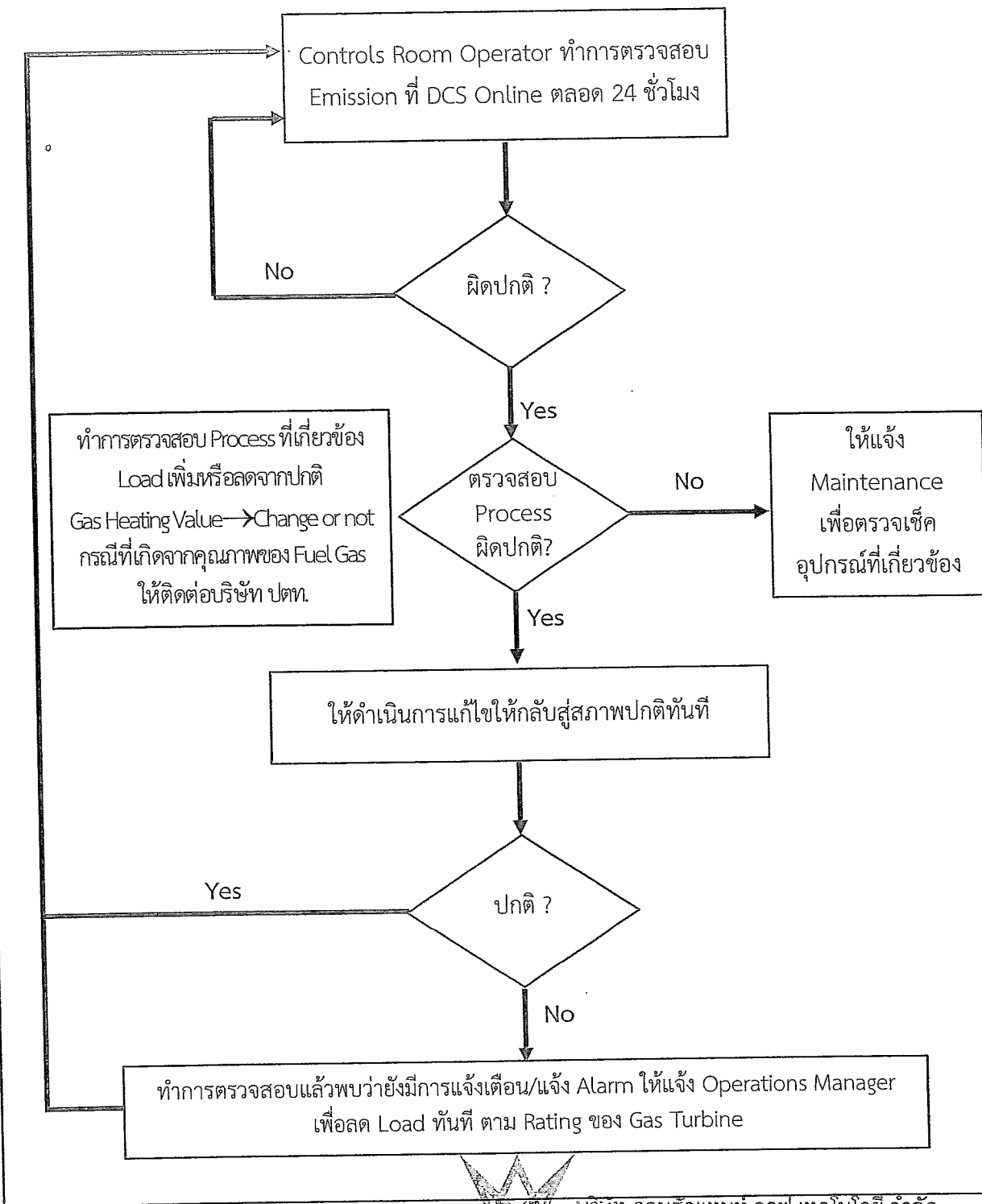
รูปที่ 1(ต่อ) Flow Chart การควบคุมและการตรวจสอบระบบสถานะทางอากาศ
