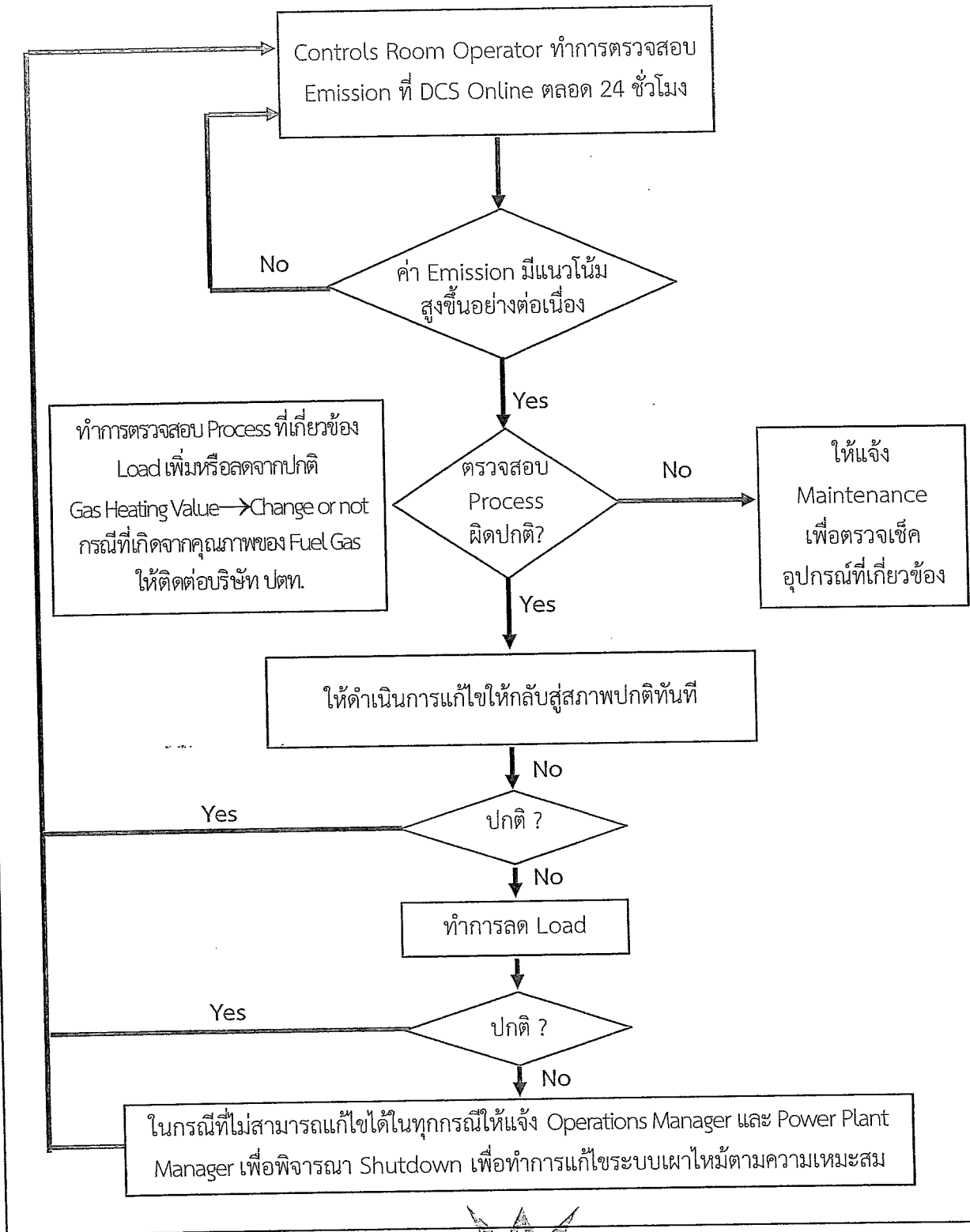
รูปที่ 1(ต่อ) Flow Chart การควบคุมและการตรวจวัดระบบเผาไหม้ทางอากาศ
