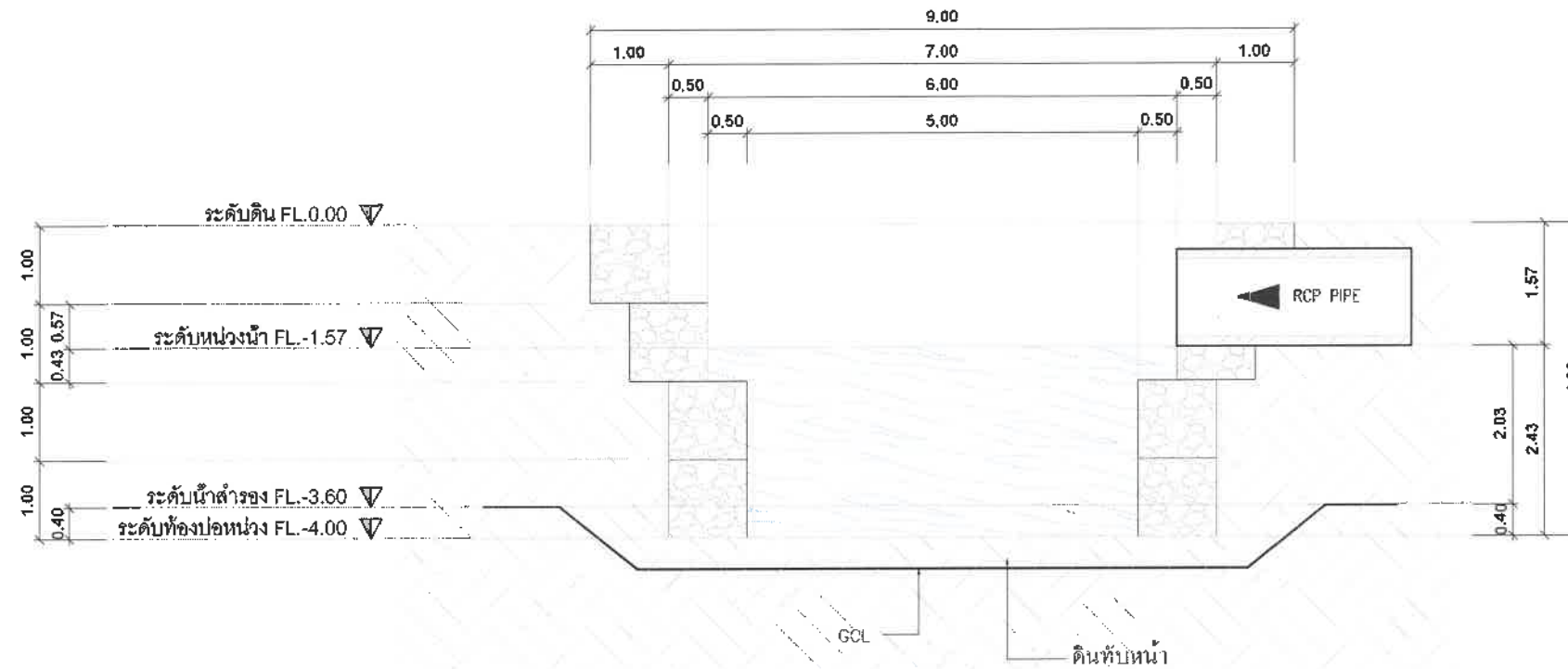
รูปตัด 1 มาตราส่วน A3 = 1:75
