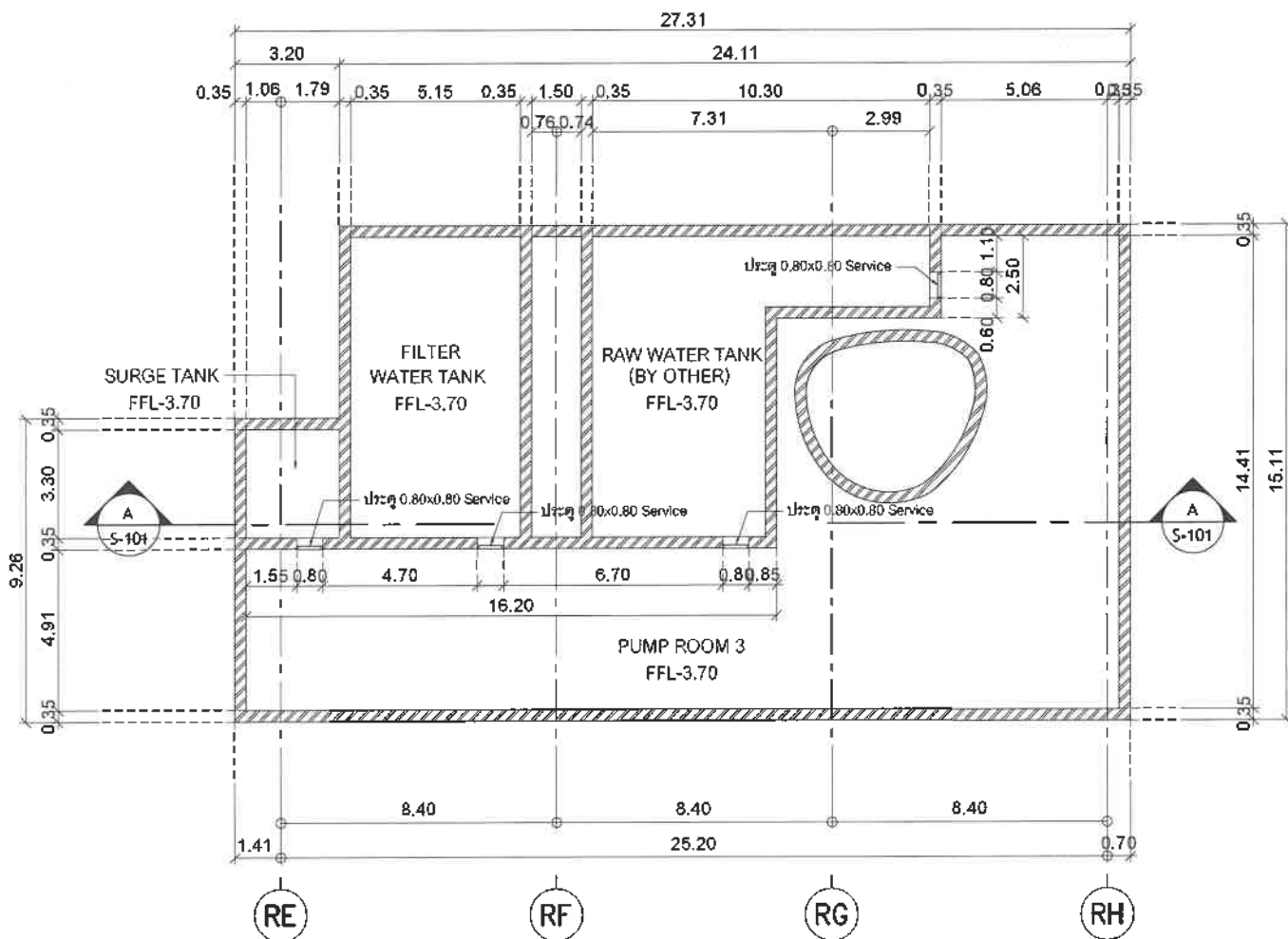
แปลนพื้นที่สระว่ายน้ำ SCALE A3 = 1:200
