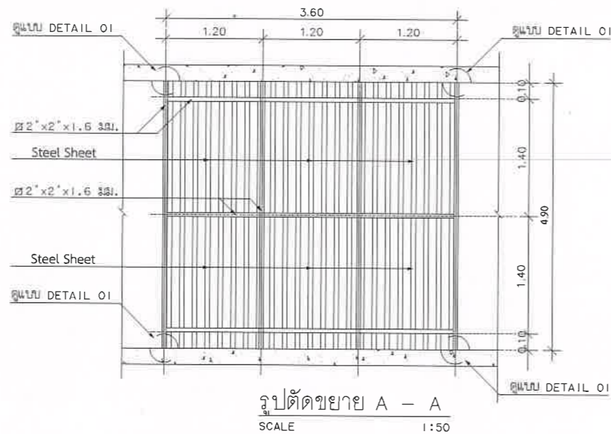
ตัวอย่างการติดตั้ง Steel Sheet
