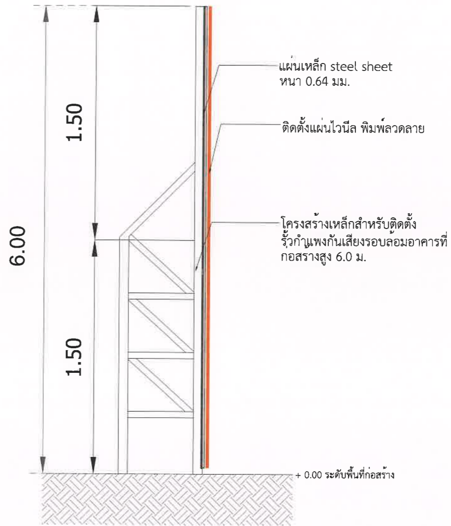
แบบขยายกำแพงกันเสียงเป็นแผ่นเหล็ก (steel sheet) สูง 6.0 เมตร ติดตั้งตามแนวเขตที่ดินของโครงการ
