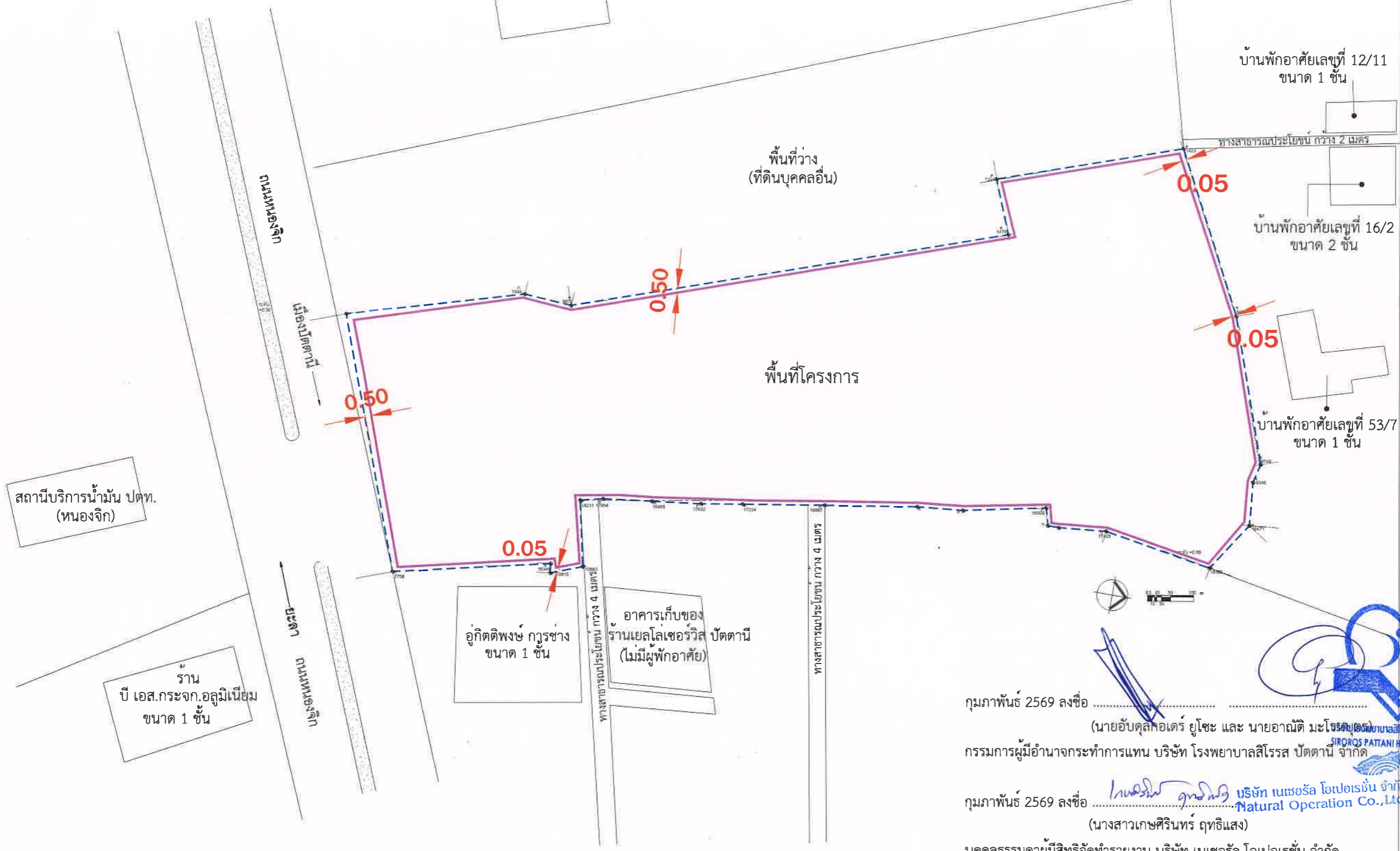
รูปที่ 10 ผังแสดงตำแหน่งแนวรั้วป้องกันผลกระทบด้านเสียงจากกิจกรรมการปรับสภาพพื้นที่โครงการ (เดือนที่ 1-3)
