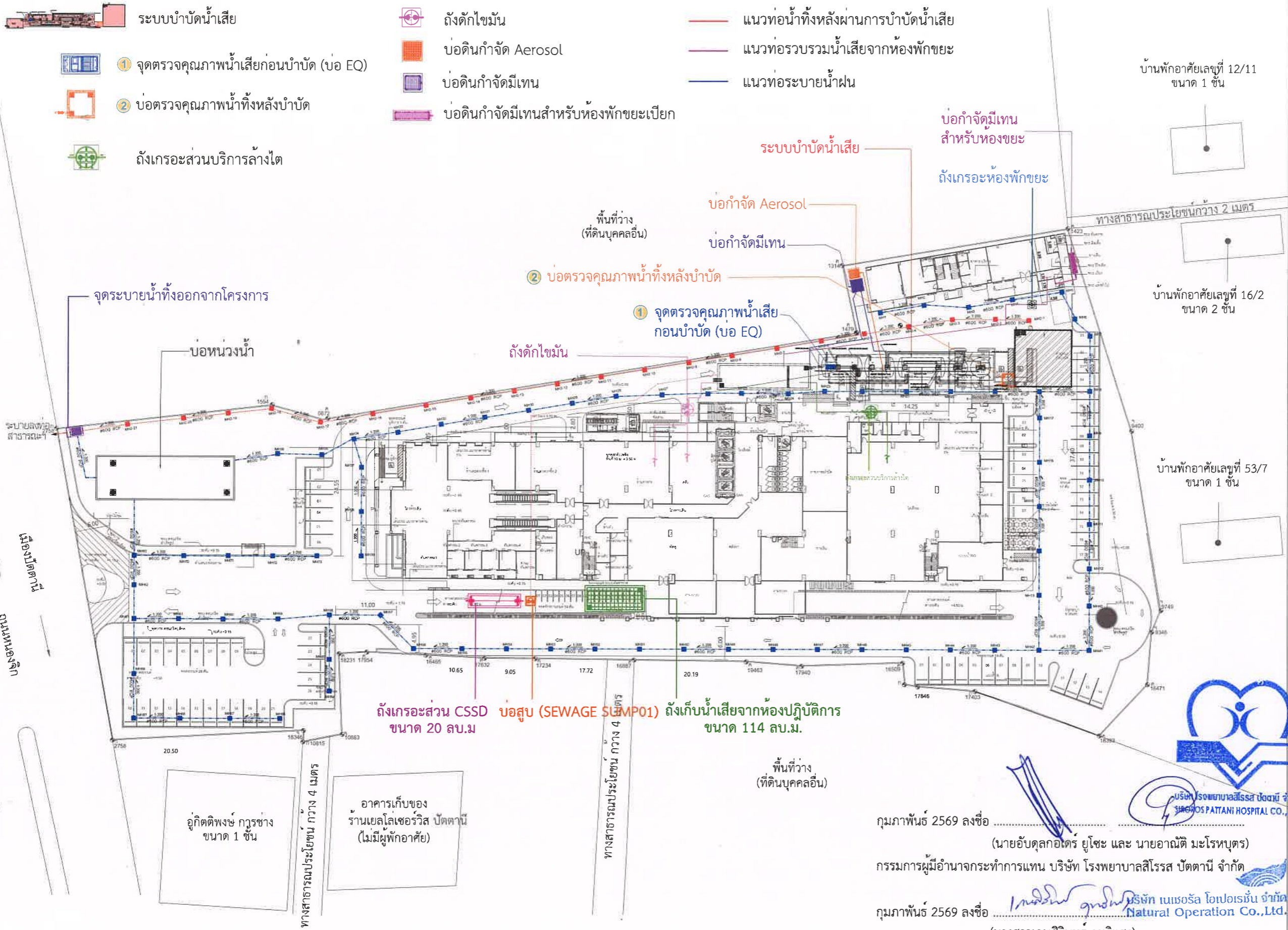
รูปที่ 3 ผังแสดงระบบสุขาภิบาล ตำแหน่งระบบบำบัดน้ำเสีย และจุดตรวจสอบคุณภาพน้ำทิ้ง (ระยะดำเนินการ)
