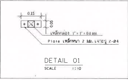
รูปที่ 11 แบบขยายการติดตั้งแผ่นเหล็ก (Steel Sheet) สูง 6 เมตร
