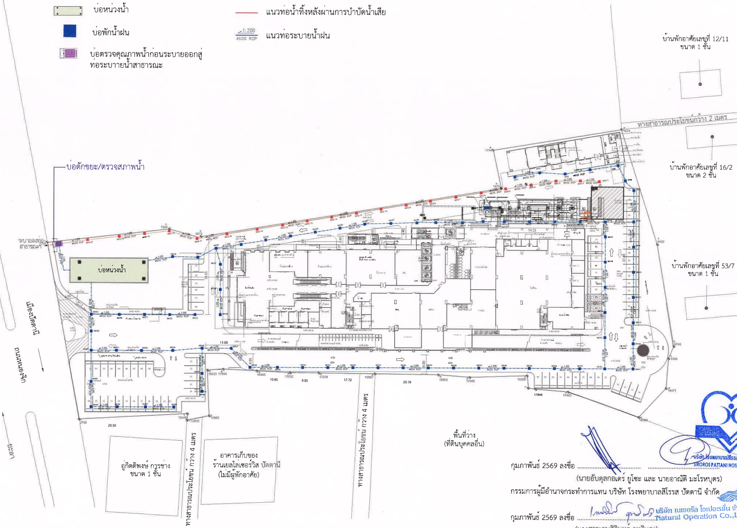
รูปที่ 4 ผังระบบระบายน้ำของโครงการ ตำแหน่งบ่อท่วงน้ำ และจุดระบายน้ำออกจากโครงการ
