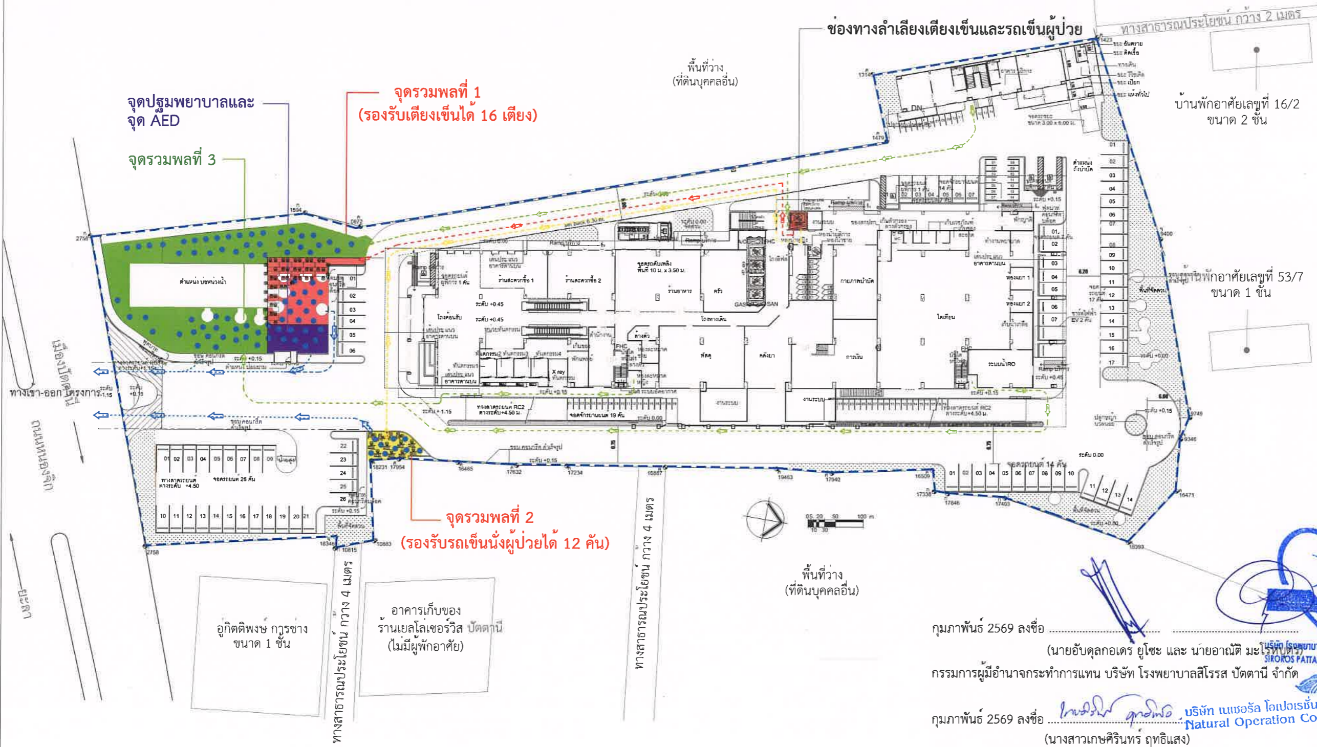
รูปที่ 8 ผังแสดงตำแหน่งจุดรวมพลของโครงการ และเส้นทางอพยพหนีไฟออกจากอาคารไปยังจุดรวมพลในโครงการ
