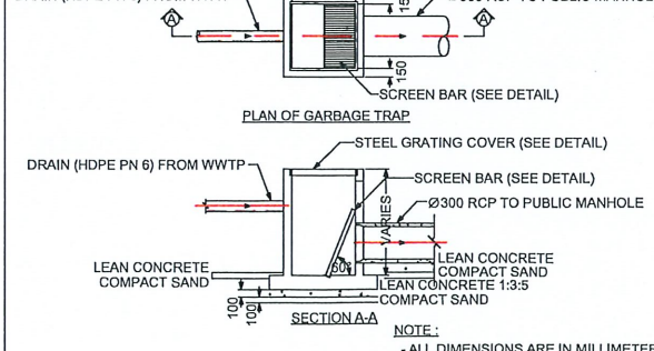
2 รายละเอียดบ่อตกขยะ NTS
