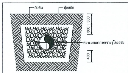
3 แบบขยายบ่อดินสำหรับกำจัดก๊าซมีเทน NTS
