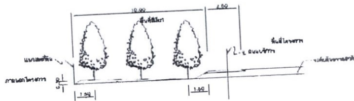
รูปตัด 2-2 การนิยามถนน
