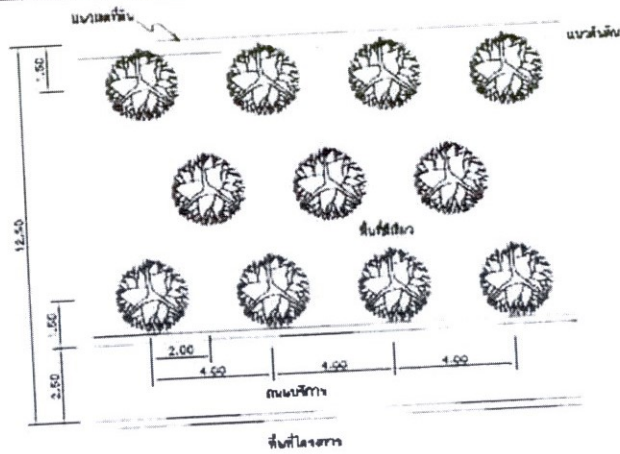
Top View 1-1 การเรียงงานชุด
