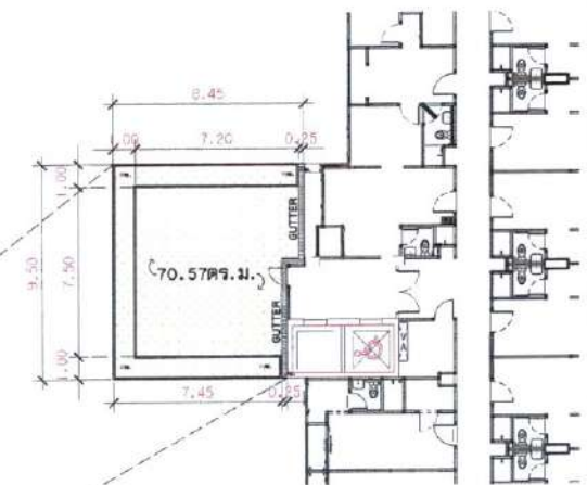
ผังแสดงพื้นที่สีเขียว ชั้น 3 มาตราส่วน 1:250
