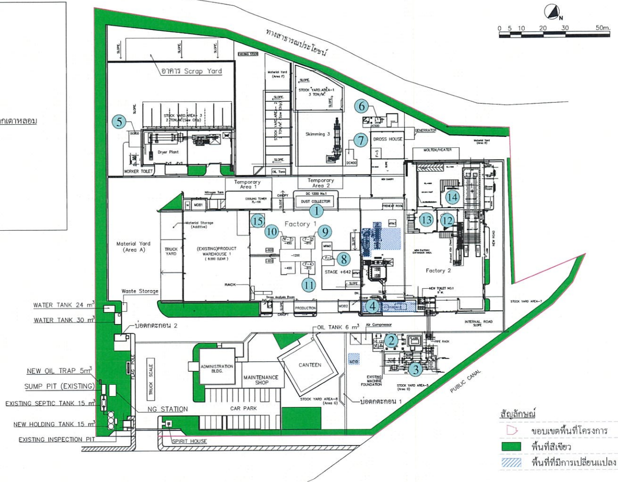
รูปที่ 8 ตำแหน่งปล่อยระบายมลพิษทางอากาศ
