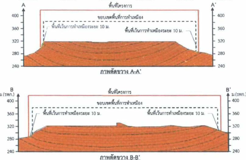
รูปที่ 4 แสดงลักษณะหน้าเหมืองและภาพตัดขวาง เมื่อสิ้นสุดการทำเหมืองปีที่ 2
