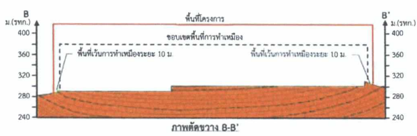
รูปที่ 7 แสดงลักษณะหน้าเหมืองและภาพตัดขวาง เมื่อสิ้นสุดการทำเหมืองปีที่ 7-9
