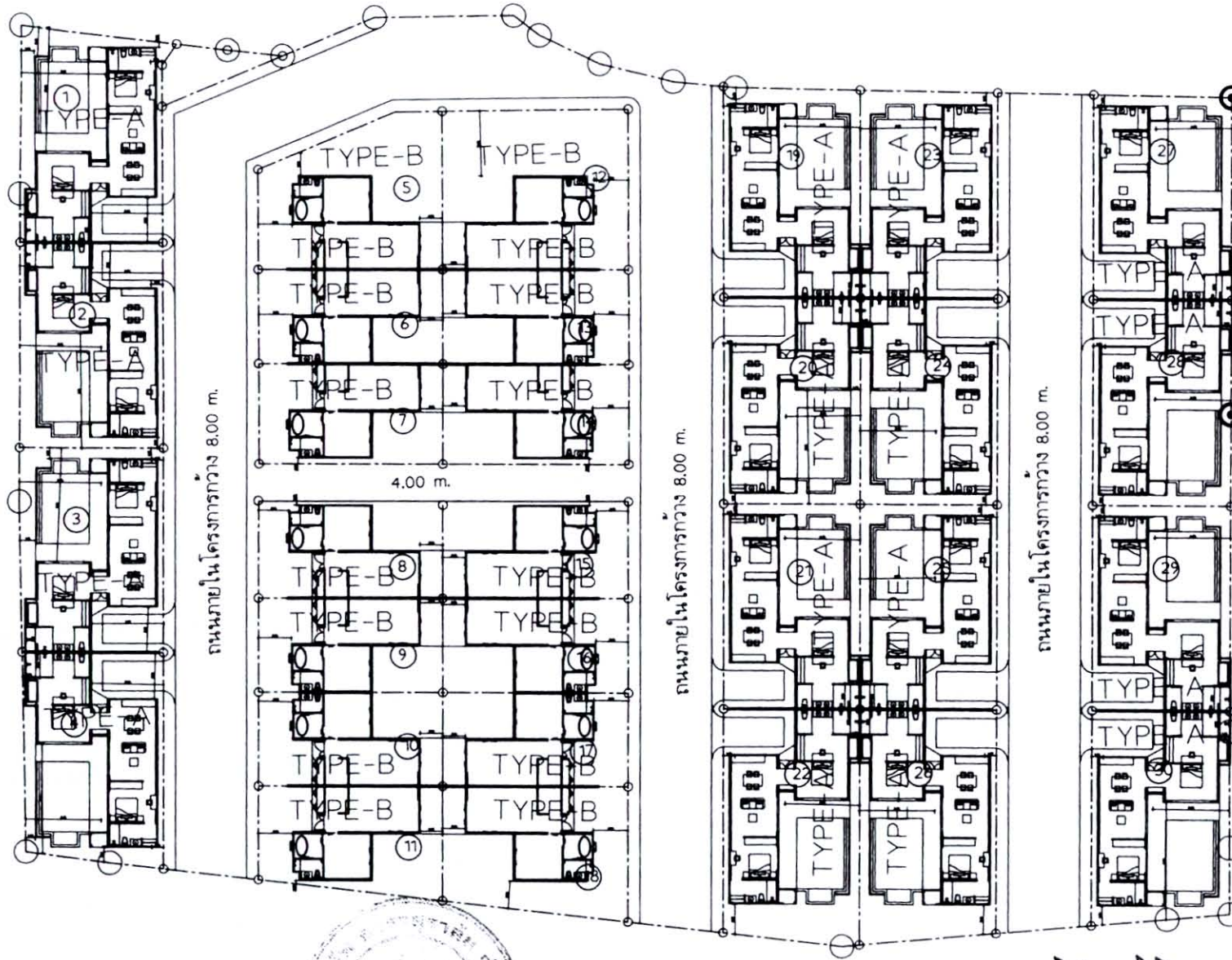
รูปที่ 2 ผังแสดงระยะถอยร่นของอาคาร
