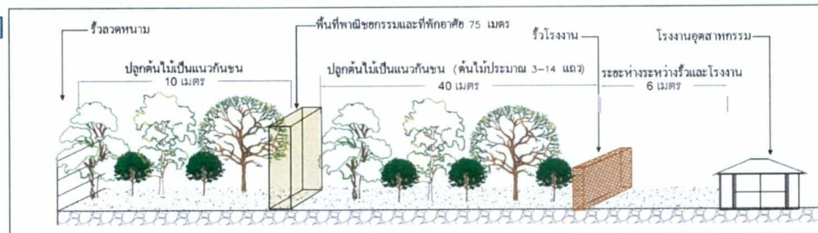
รูปที่ 6 แสดงแนวกันชนบริเวณทางด้านทิศตะวันตกของโครงการ
