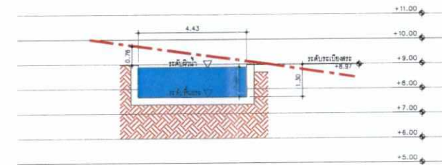
BUILDING SWIMMING POOL 2 (+8.97) (พื้นที่ความชื้นเฉลี่ยร้อยละ 13.72)
