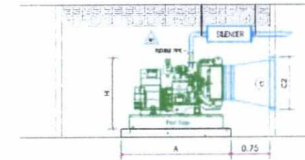
แบบขยายการติดตั้ง GENERATOR 1,000 kVA
