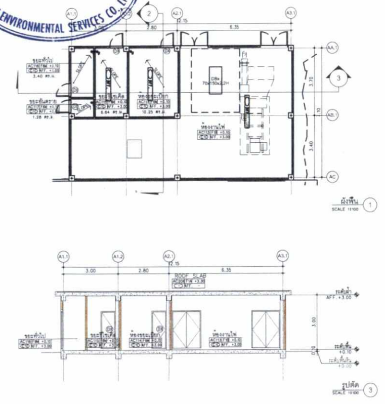
แบบขยายห้องขยะ
