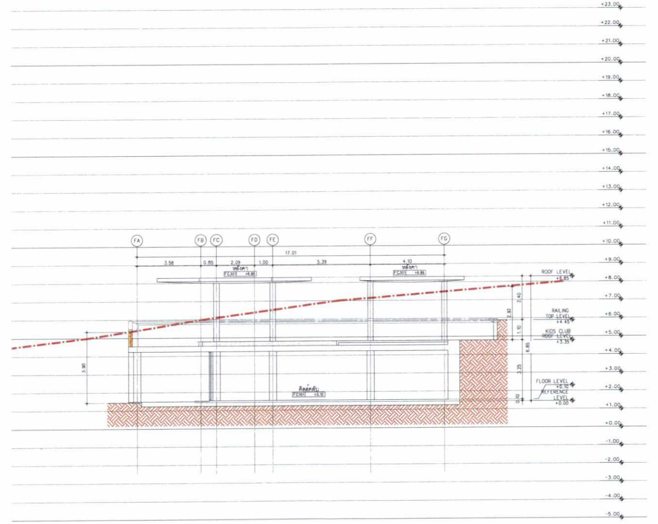
BUILDING F (+7.00) (พื้นที่ความชันเฉลี่ยร้อยละ 12.08)
