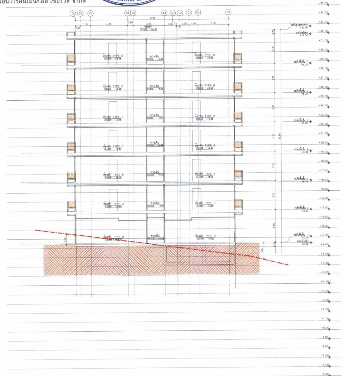
BUILDING C (+9.40) (พื้นที่ความชันเฉลี่ยร้อยละ 12.93)
