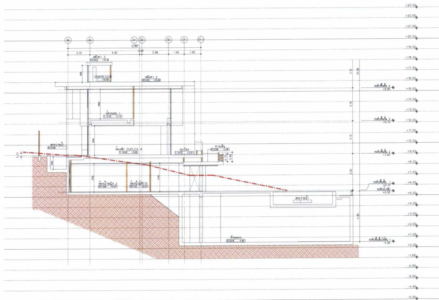
BUILDING D (+5.40) (พื้นที่ความชันเฉลี่ยร้อยละ 16.48)
