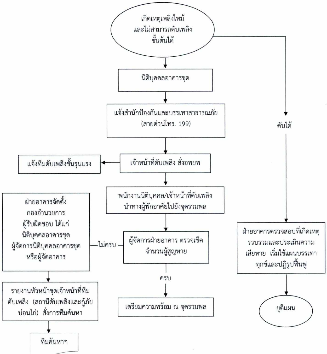
รูปที่ 5 แผนภาพแสดงการดับเพลิงและการอพยพ
