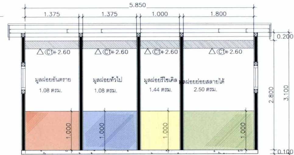
รูปตัด B-B SCALE 1:40
