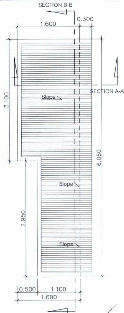
แปลนหลังคา อาคารพักขยะ SCALE 1:40
