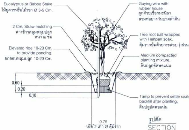
รูปตัด SECTION
