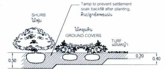
รูปตัด SECTION
