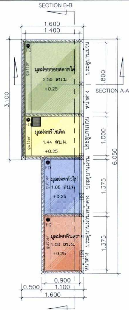
แปลนพื้น อาคารพักขยะ SCALE 1:40
