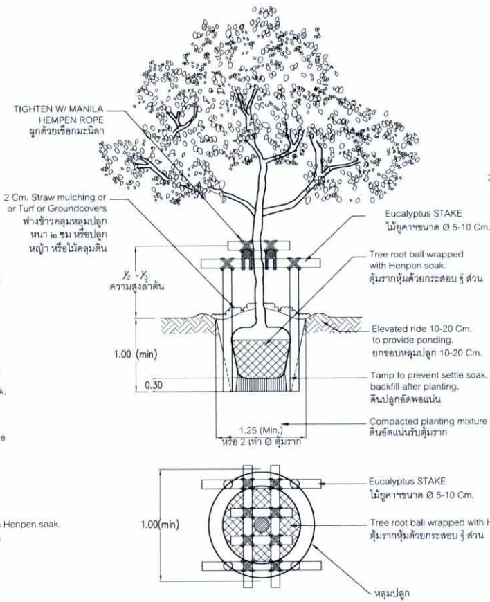
รูปที่ 18 แบบขยายการปลูกต้นไม้ของโครงการ
