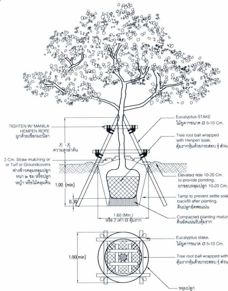
รูปที่ 18 แบบขยายการปลูกต้นไม้ของโครงการ
