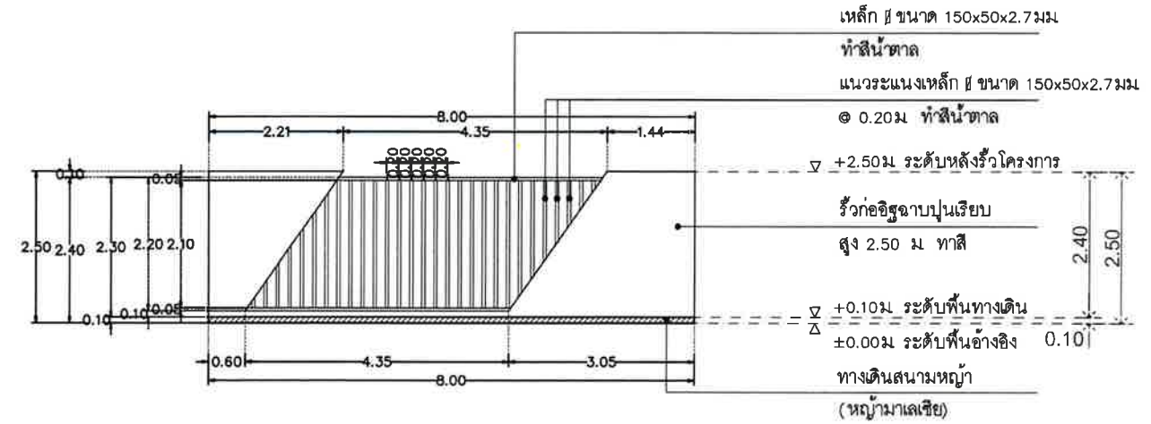
แบบขยายรูปด้านหน้าโครงการ มาตรฐาน 1:50 0 1 2 5 เมตร
