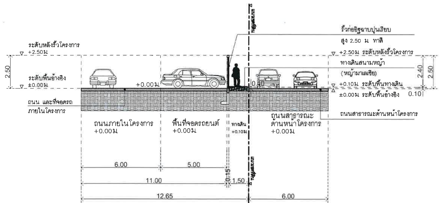
แบบขยายรูปตัดทางเดินด้านหน้าโครงการ มาตรฐาน 1:75 0 1 2 5 เมตร
