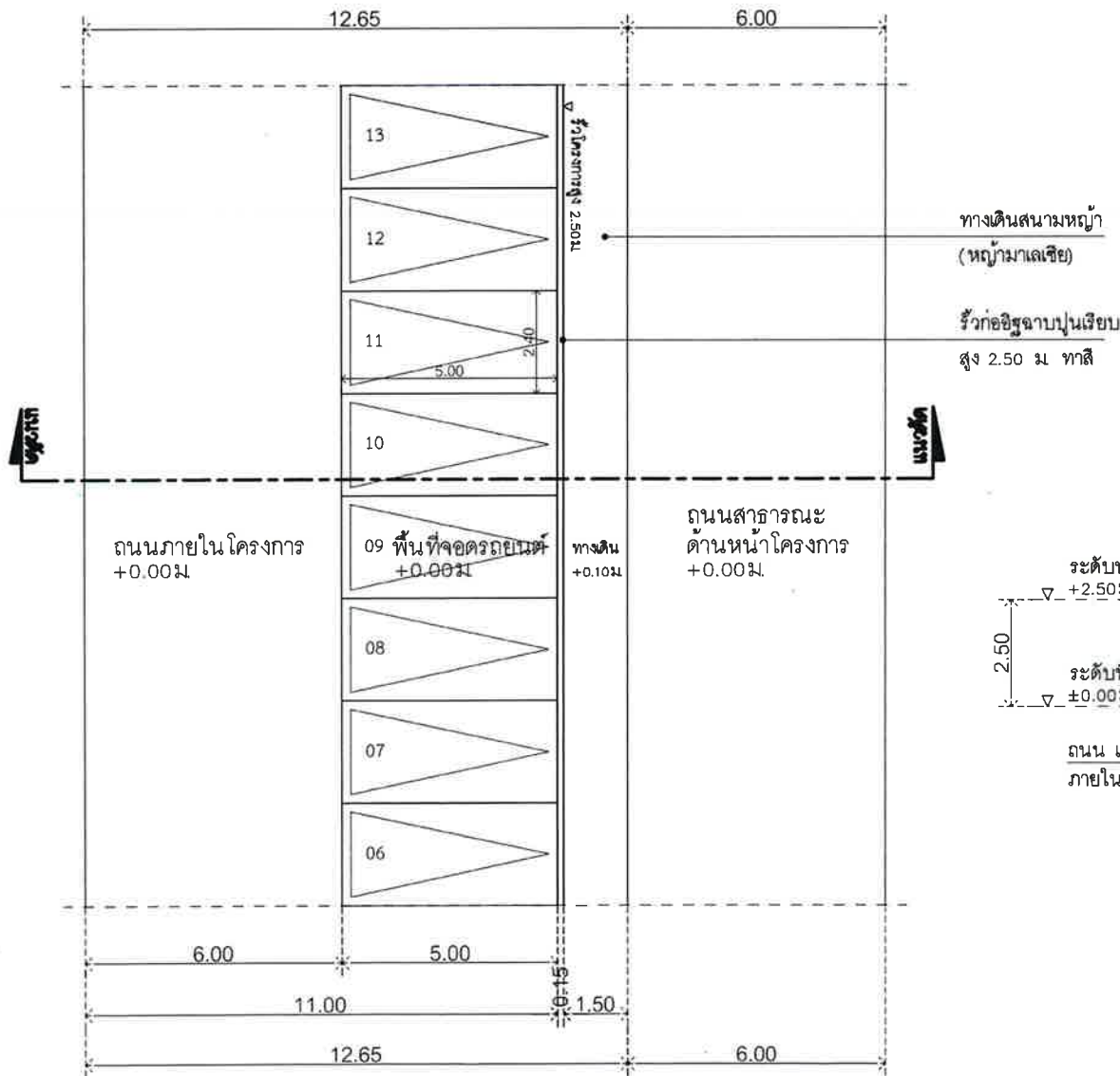
แบบขยายแปลนทางเดินด้านหน้าโครงการ มาตรฐาน 1:75 0 1 2 5 เมตร
