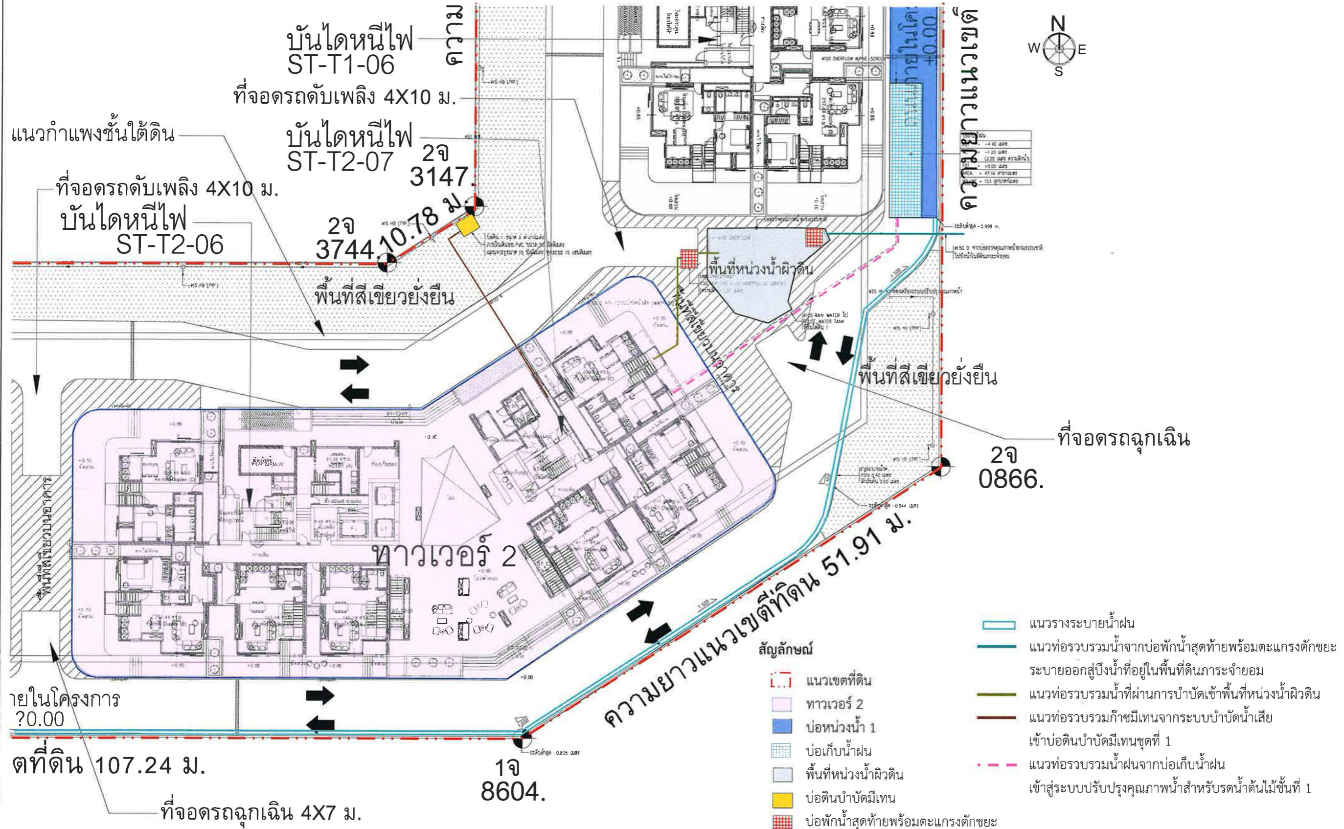
รูปที่ 8 ผังระบบระบายน้ำฝน และน้ำเสียของโครงการ (ส่วนที่ 2)
