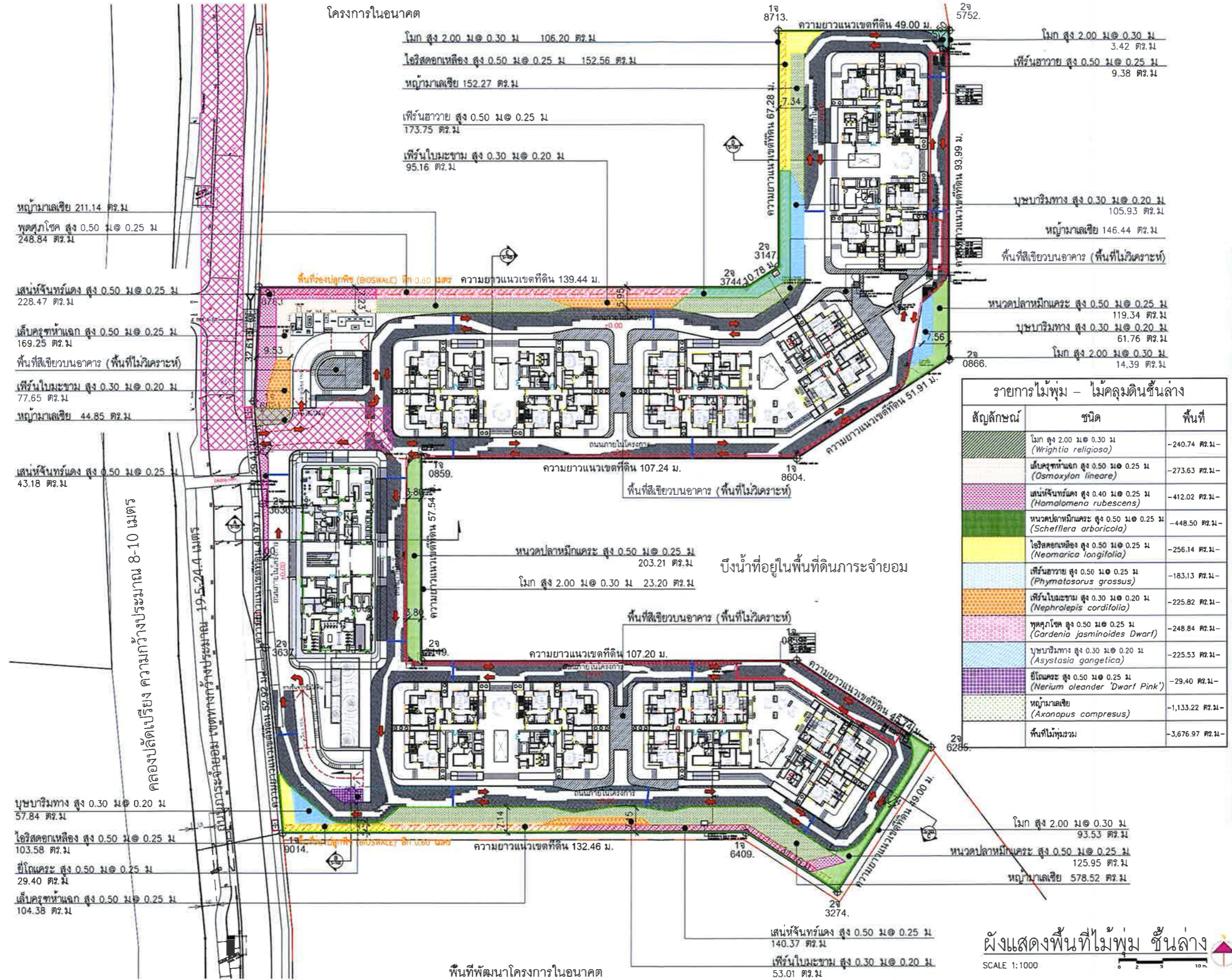
รูปที่ ผ.1-4 ผังแสดงการปลูกไม้พุ่มและไม้คลุมดินบริเวณชั้นที่ 1 ของโครงการ
