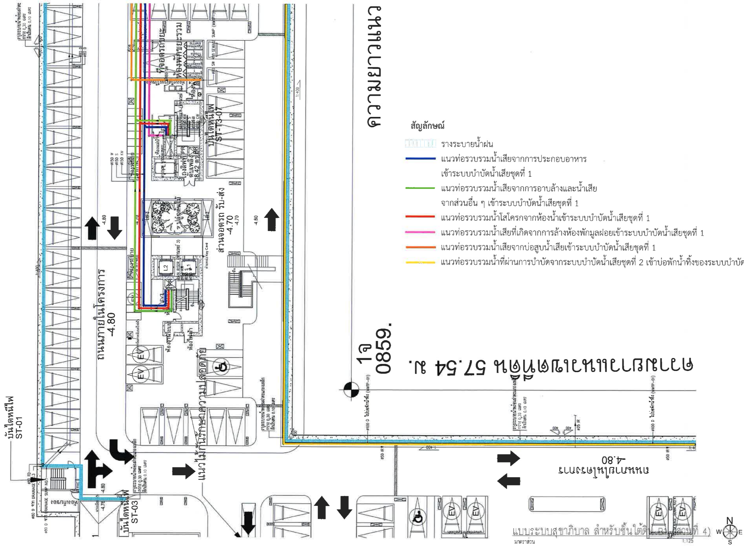
รูปที่ 24 ผังระบบระบายน้ำฝน และน้ำเสียชั้นใต้ดิน B1 (ส่วนที่ 4)
