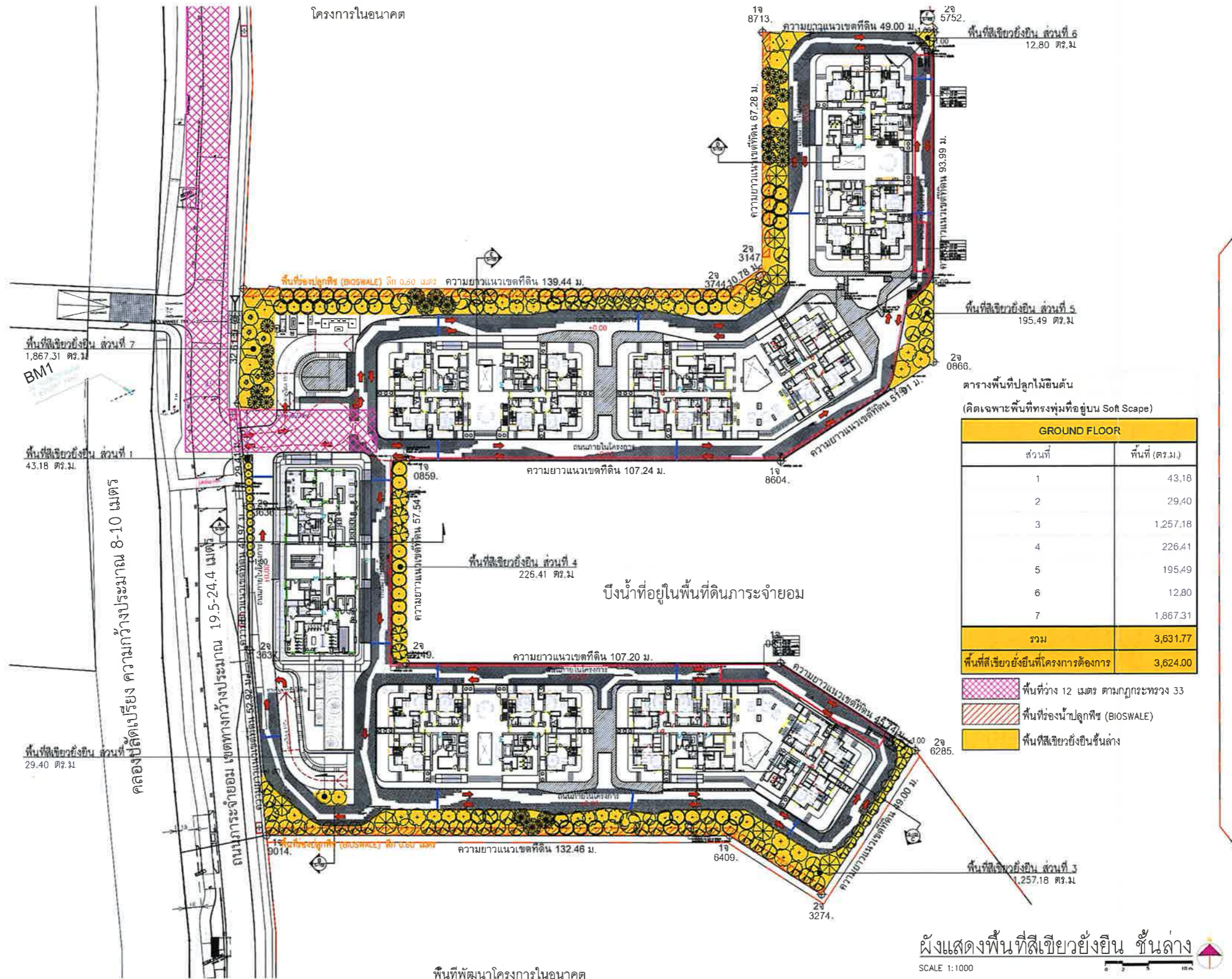
รูปที่ ผ.1-3 ผังแสดงการปลูกไม้ยืนต้น และระบบสาธารณูปโภคบริเวณชั้นที่ 1 ของโครงการ
