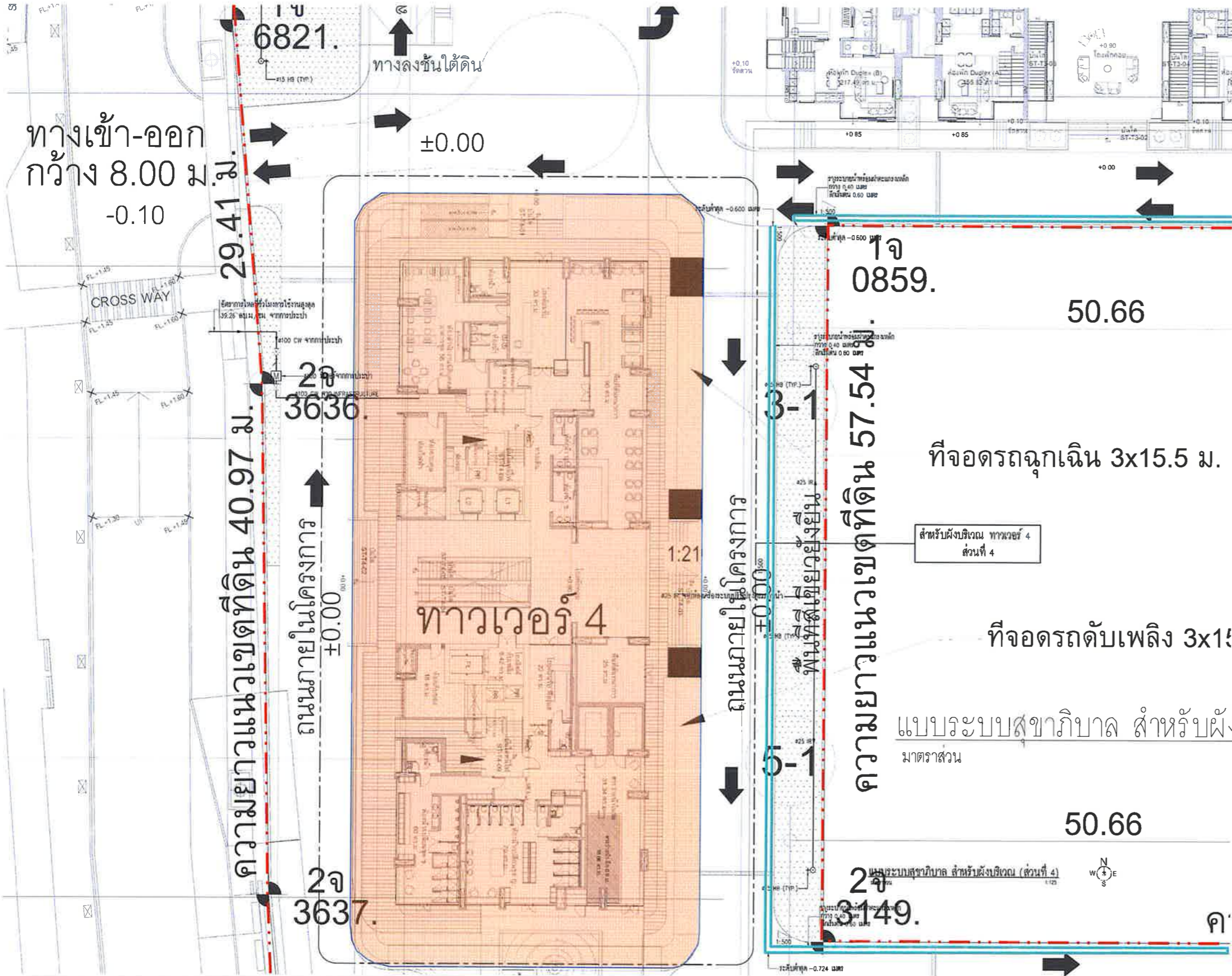
รูปที่ 10 ผังระบบระบายน้ำฝน และน้ำเสียของโครงการ (ส่วนที่ 4)
