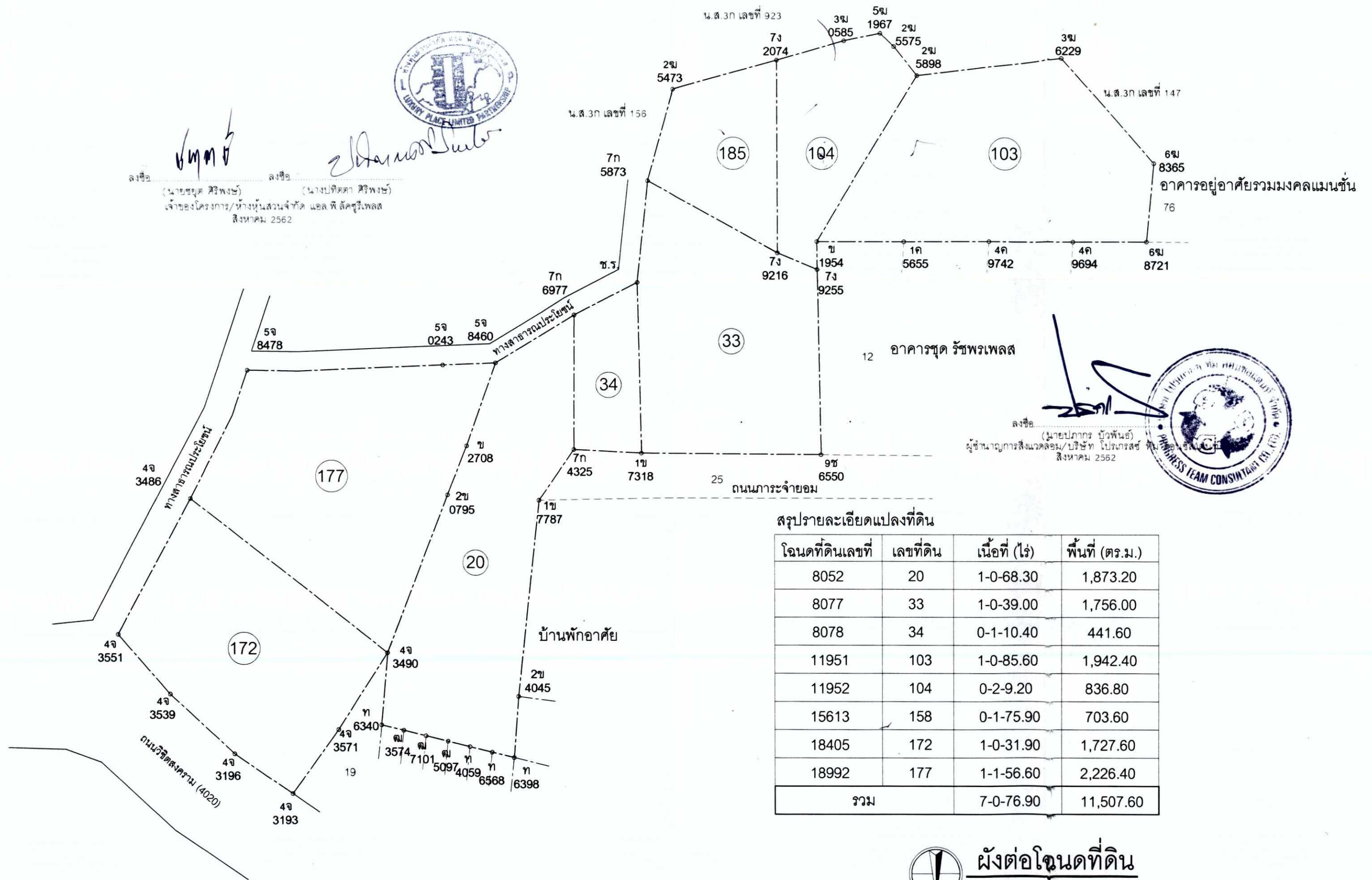
รูปที่ 1 ผังต่อโฉนดที่ดินของโครงการ
