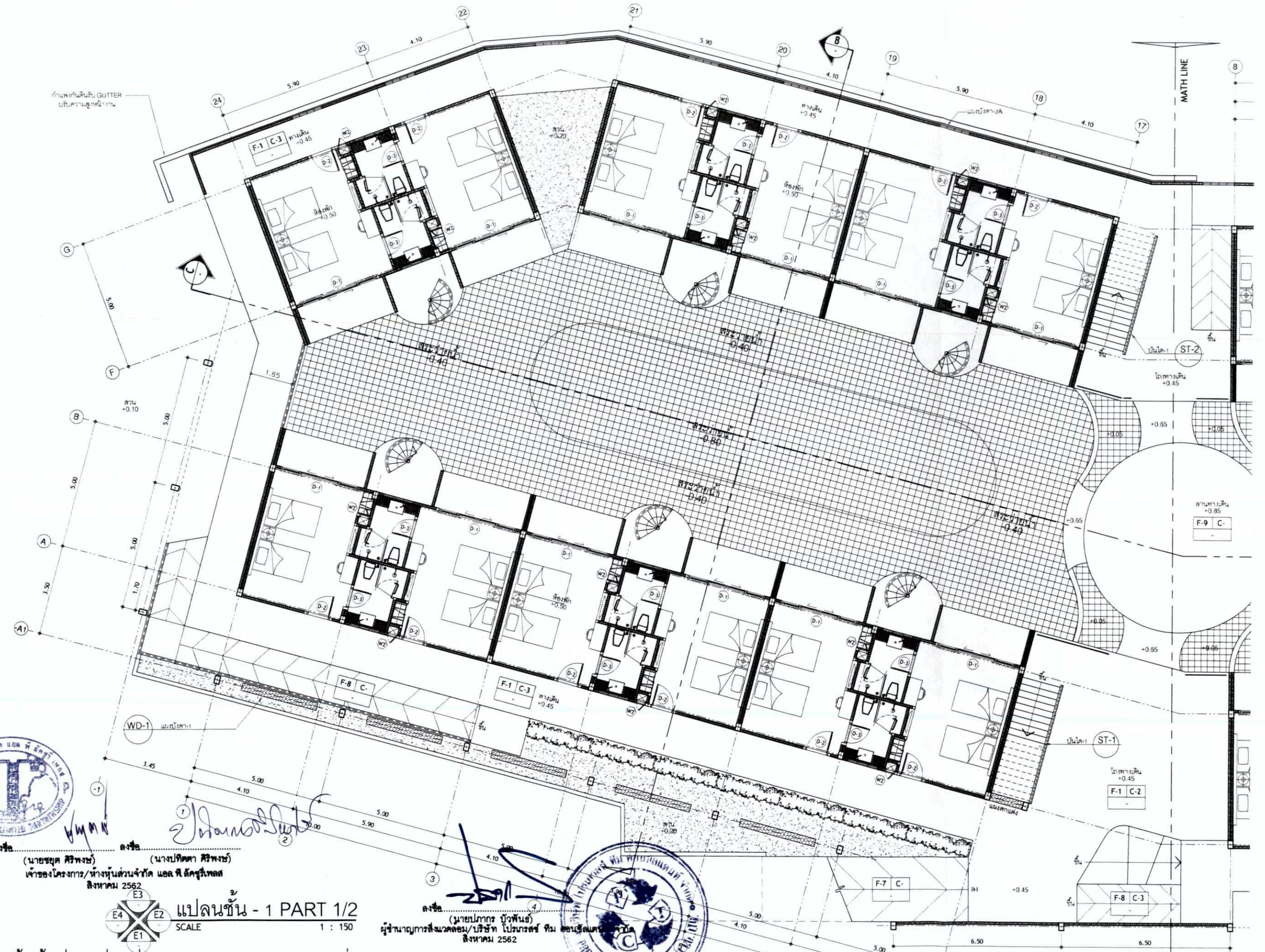
รูปที่ 16 แปลนพื้นที่ 1 (ส่วนที่ 1/2) ของอาคาร 3 (อาคารส่วนขยาย)
