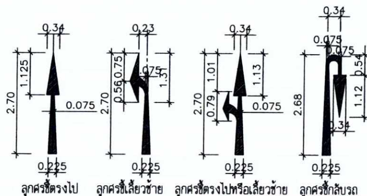
แบบขยายสัญลักษณ์ทิศทางการจราจร มาตราส่วน 1 : 100
