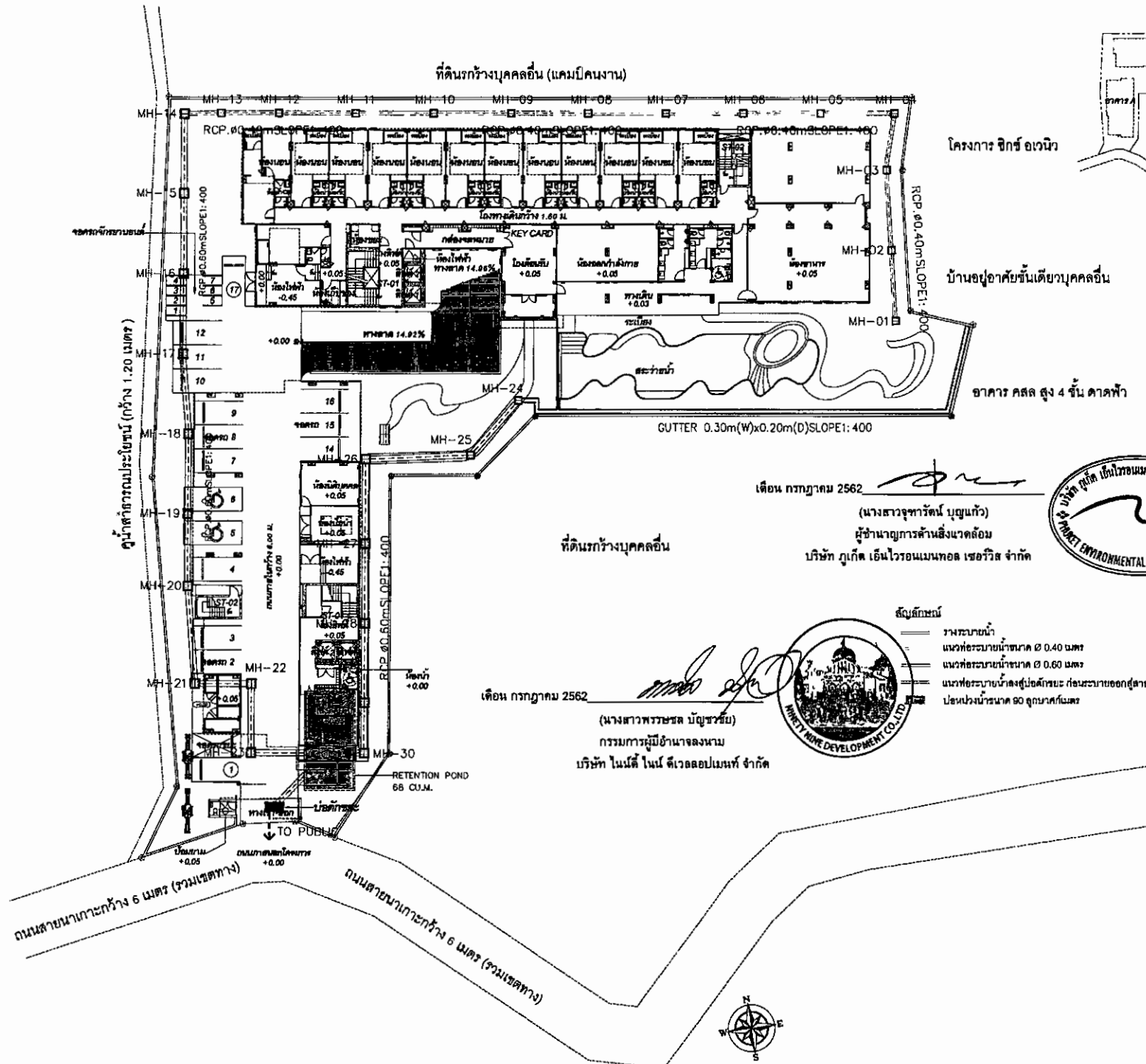
รูปที่ 8 หวังระบบระบายน้ำฝนของโครงการ
