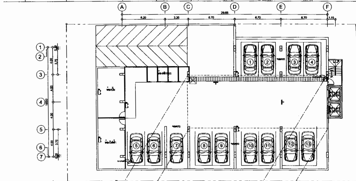
รูปที่ 12 ผังแสดงตำแหน่งจุดติดตั้งระบบโทรทัศน์วงจรปิด
