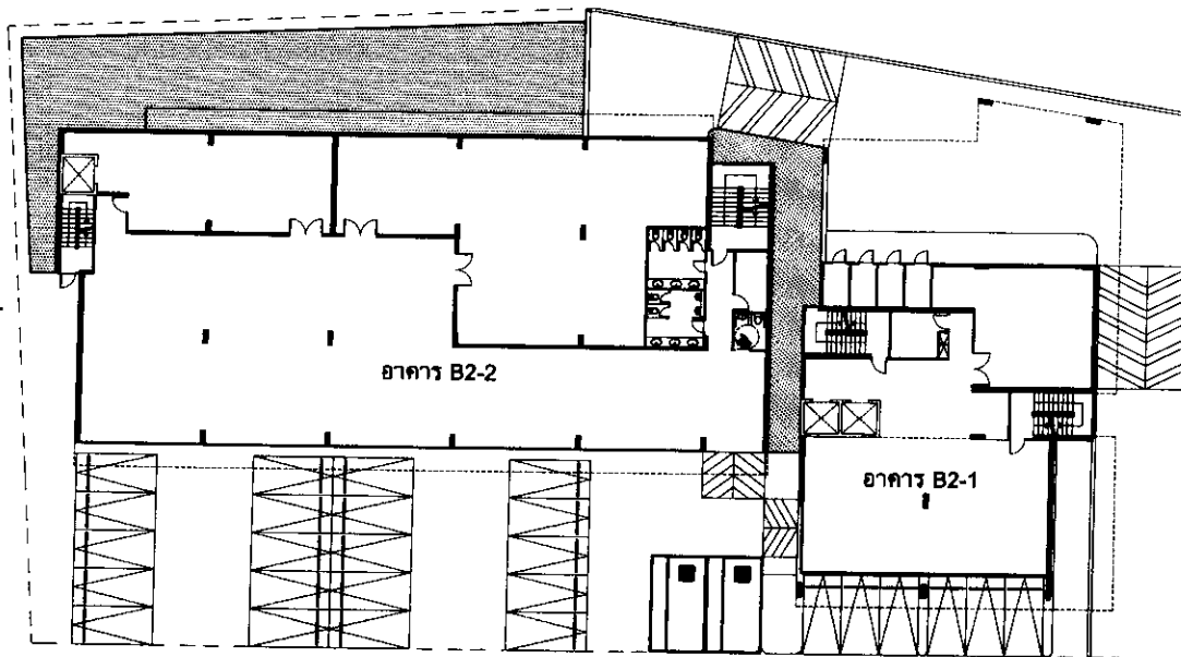
แปลนพื้นที่ 1
