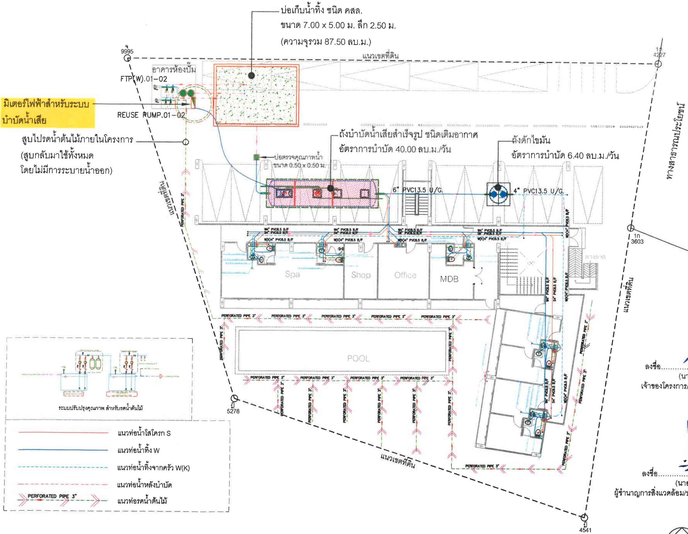
รูปที่ 7 ผังระบบบำบัดน้ำเสียของโครงการ
