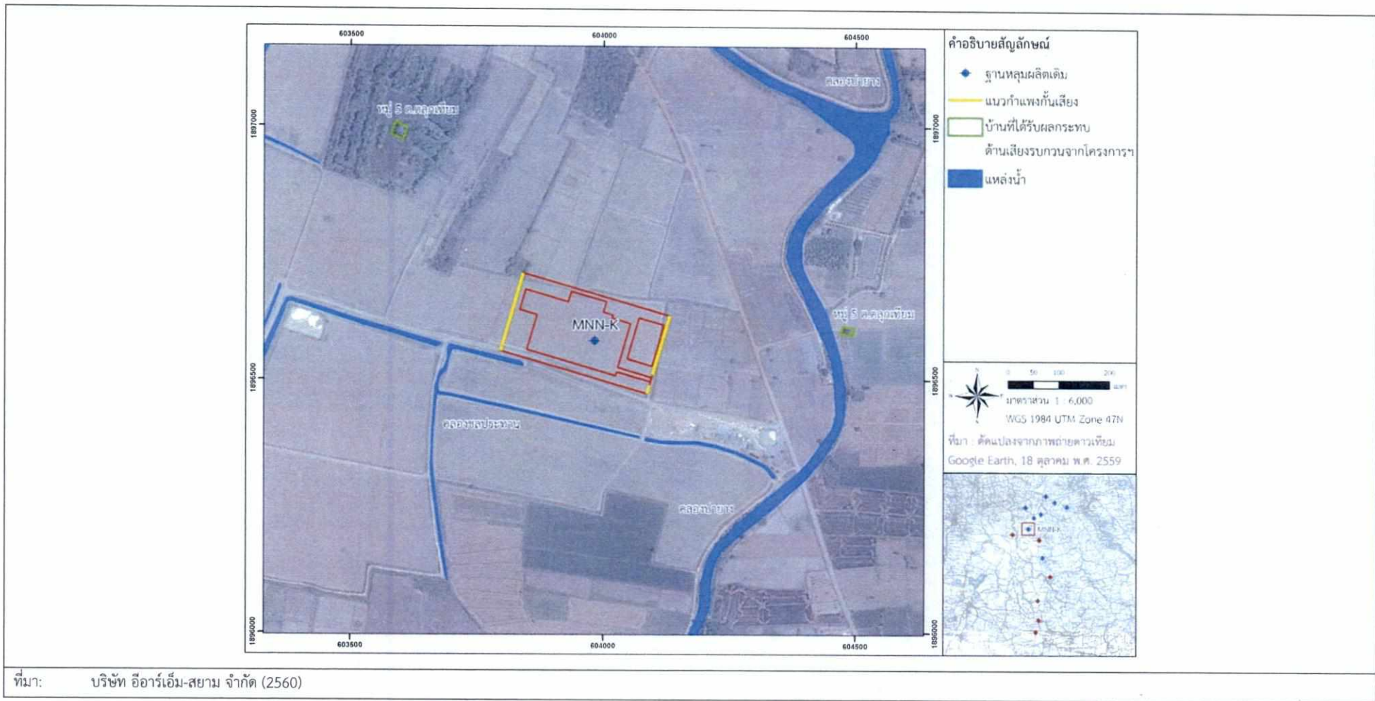
รูปที่ 2 แนวการติดตั้งกำแพงกันเสียงบริเวณขอบฐานหลุมผลิตแม่น้ำน่าน-เค (MNN-K) ในระยะก่อสร้างและติดตั้ง
