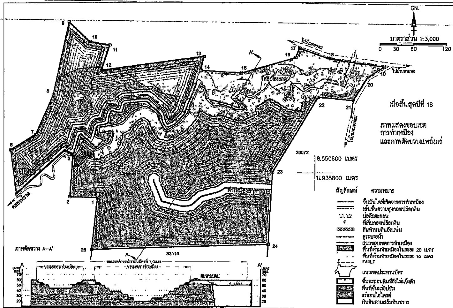
รูปที่ 10: ภาพแสดงขอบเขตการทำเหมือง และภาพตัดขวางแหล่งแร่ เมื่อสิ้นสุดปีที่ 18
