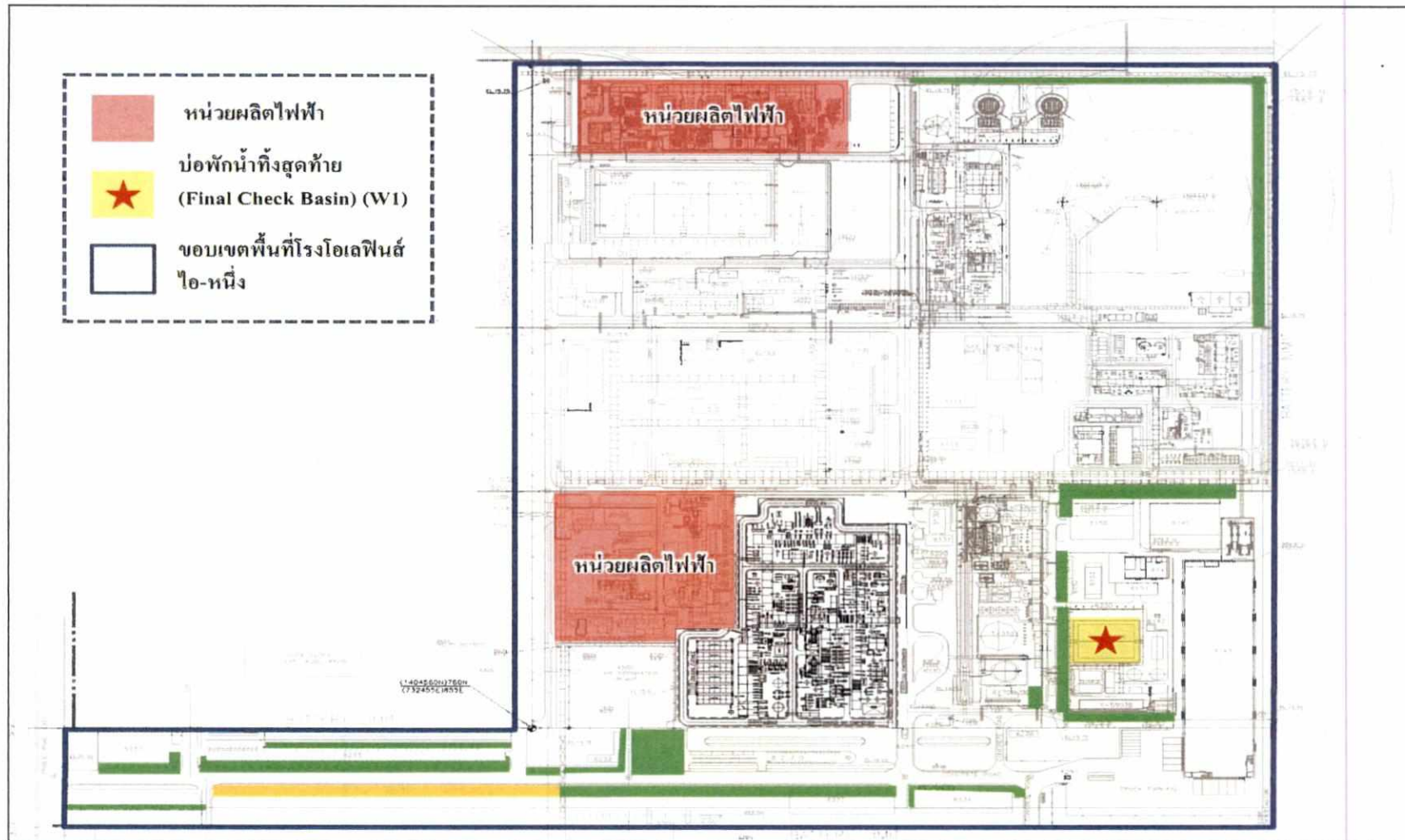
รูปที่ 4 จุดเก็บตัวอย่างน้ำทิ้งบริเวณบ่อพักน้ำทิ้งสุดท้ายของโรงโอดเลฟินส์
