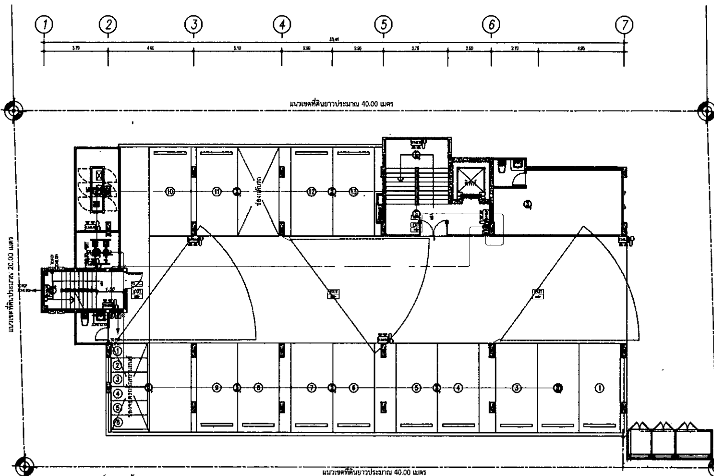
รูปที่ 12 แสดงแปลนระบบอัคคีภัยและความปลอดภัยชั้นที่ 1
