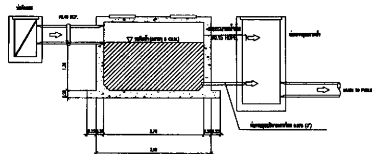
รูปตัด แนว ยาว
