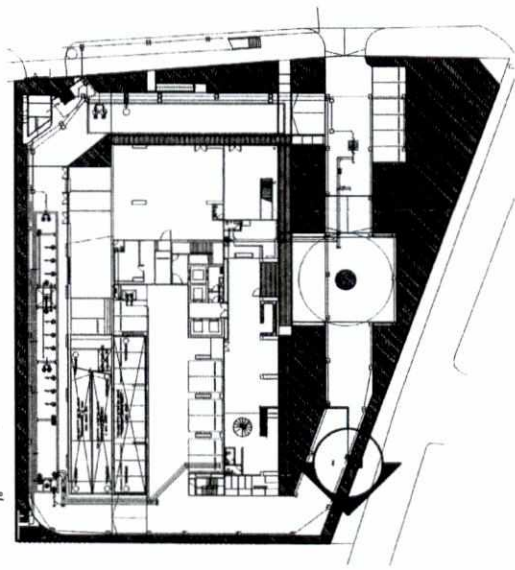
ผังอ้างอิงชั้น 1
