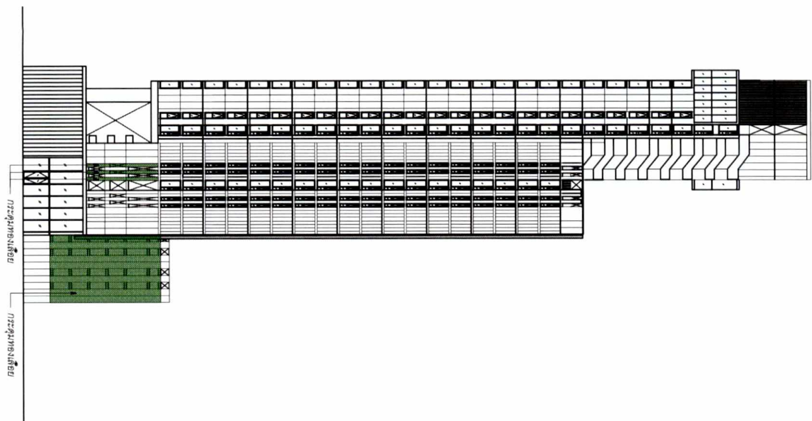
รูปด้านแสดงตำแหน่งไม้เลื้อยฝั่งทิศตะวันตก
