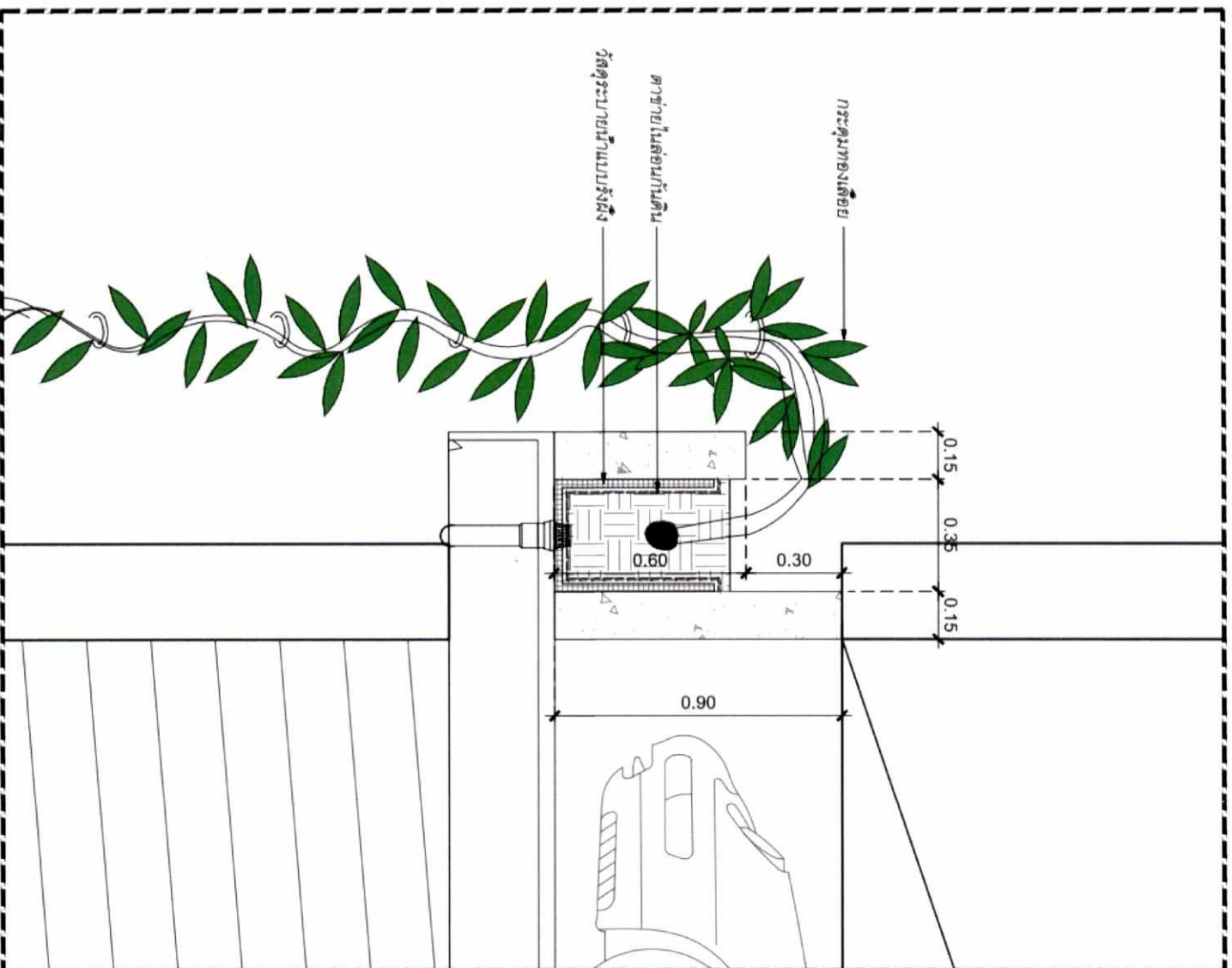
รูปตัดขยายแสดงพื้นที่วางกะละมัง มาตราส่วน 1:20
