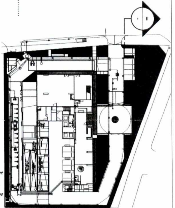
ผังอ้างอิงชั้น 1
