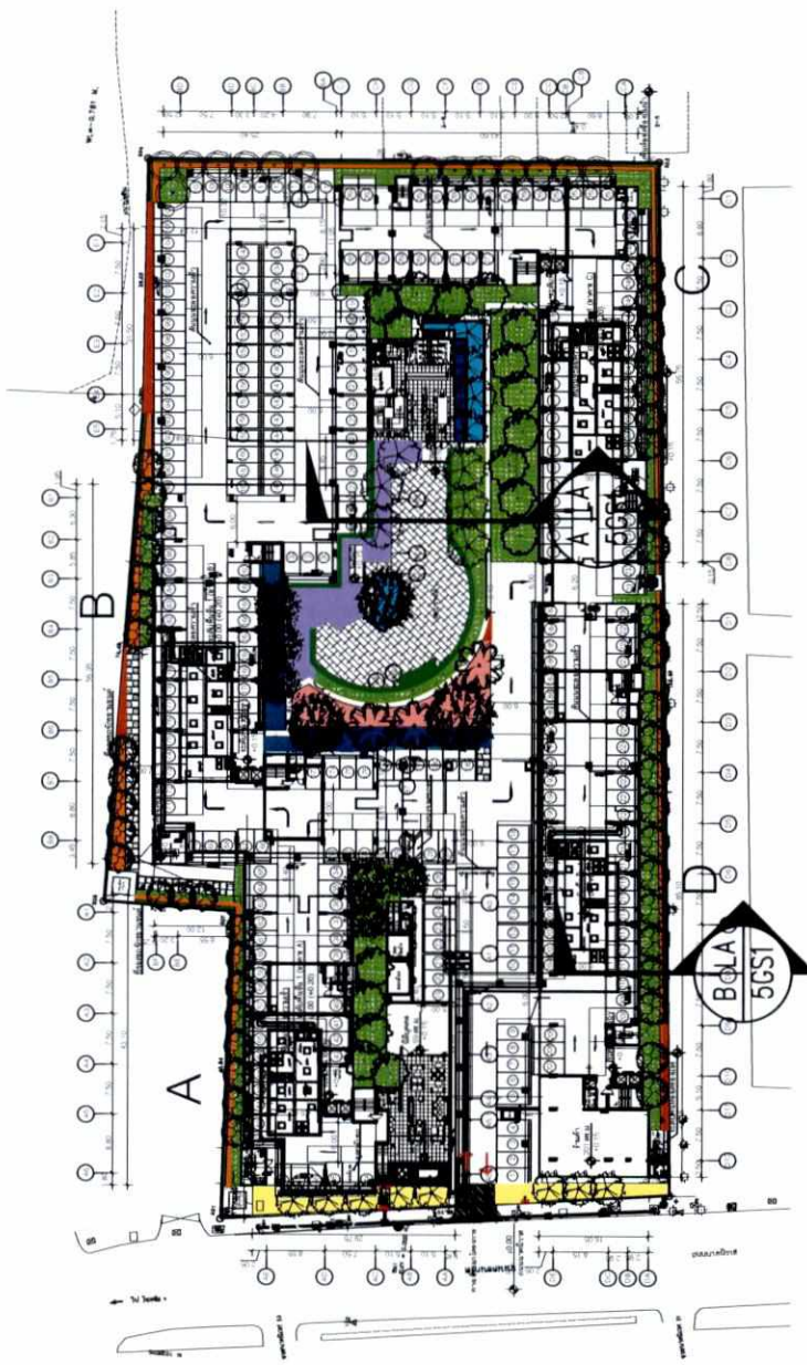
ผังแสดงแนวตัดพื้นที่สีเขียวชั้นล่าง SCALE A3=1:NTS
