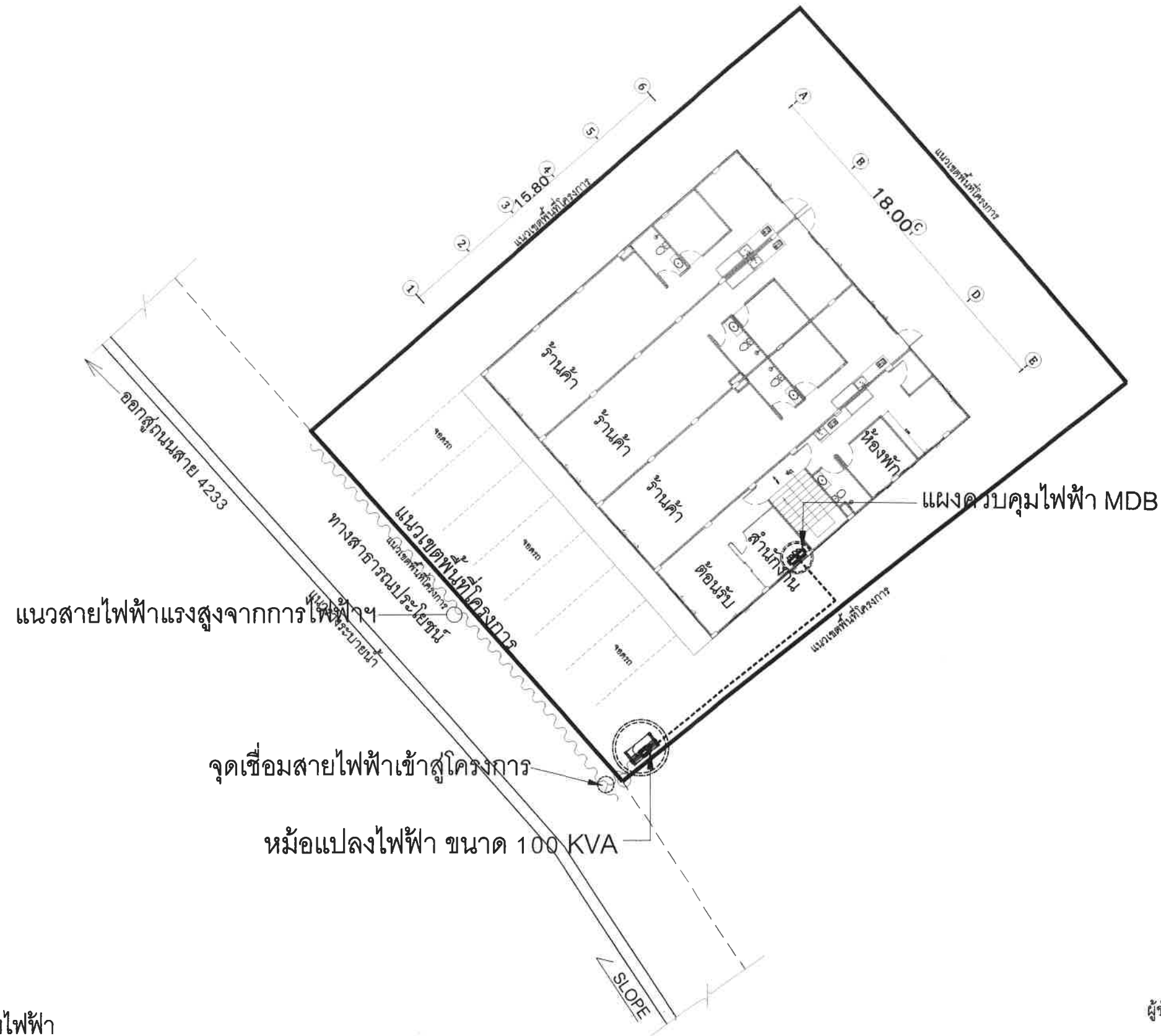
รูปที่ 7 ผังระบบไฟฟ้าของโครงการ
