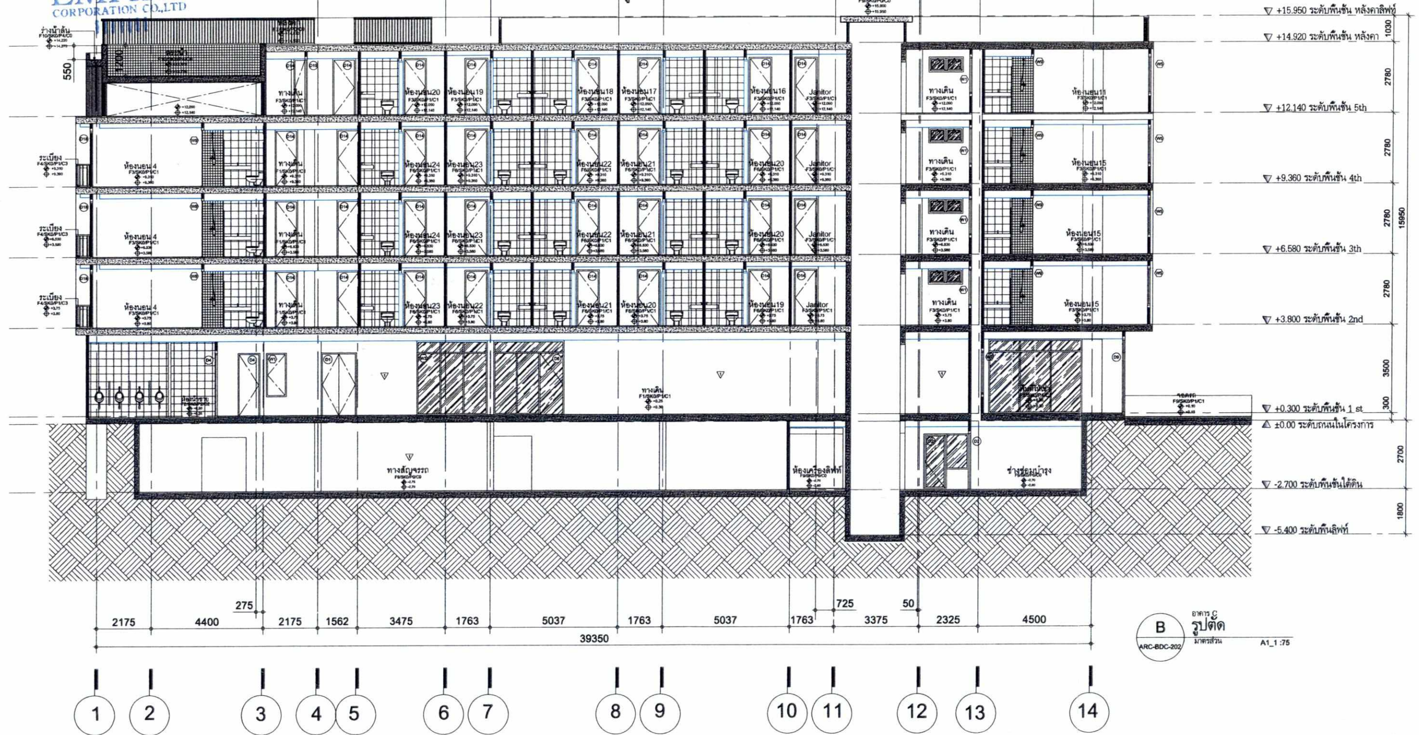
รูปที่ 31 รูปตัด B อาคาร C
