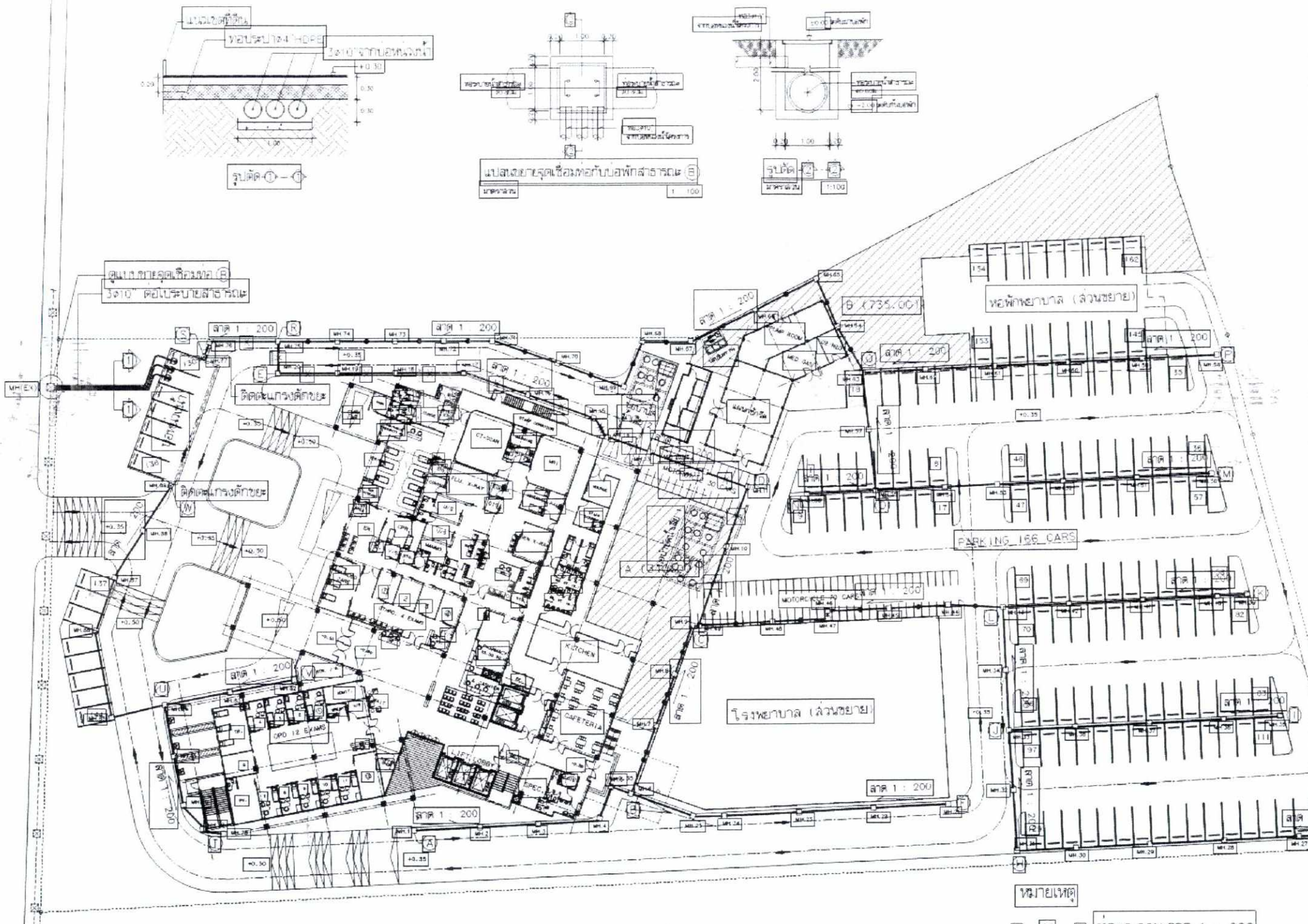
รูปที่ 6 แบบแสดงระบบระบายน้ำฝนของโครงการ
