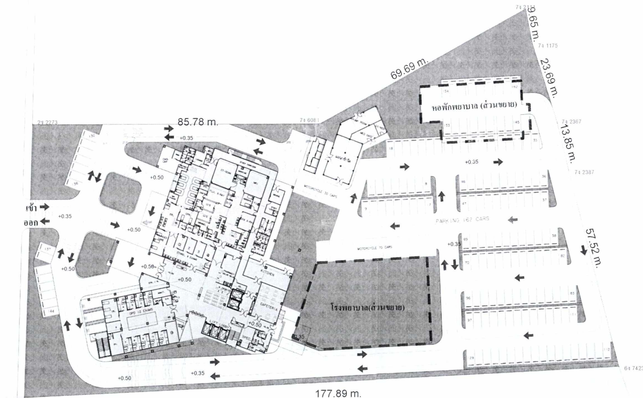
รูปที่ 13 แสดงแนวเส้นทางจราจรภายในโครงการ
