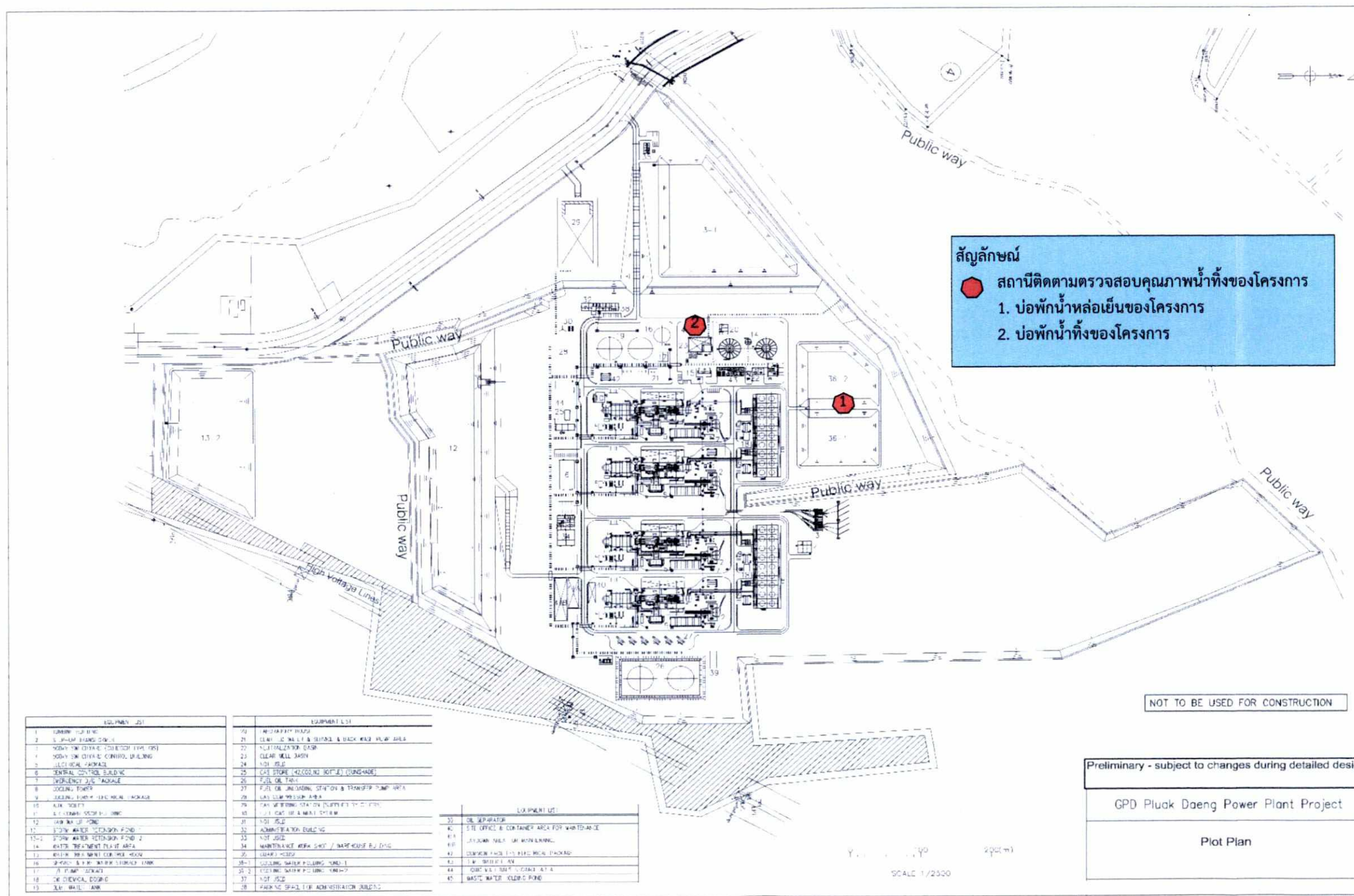
รูปที่ 3 : สถานีติดตามตรวจสอบคุณภาพน้ำทั้งของโครงการ
