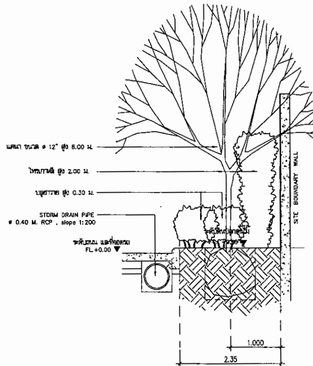
รูปตัด A2 ขนาดเส้น 1:50
