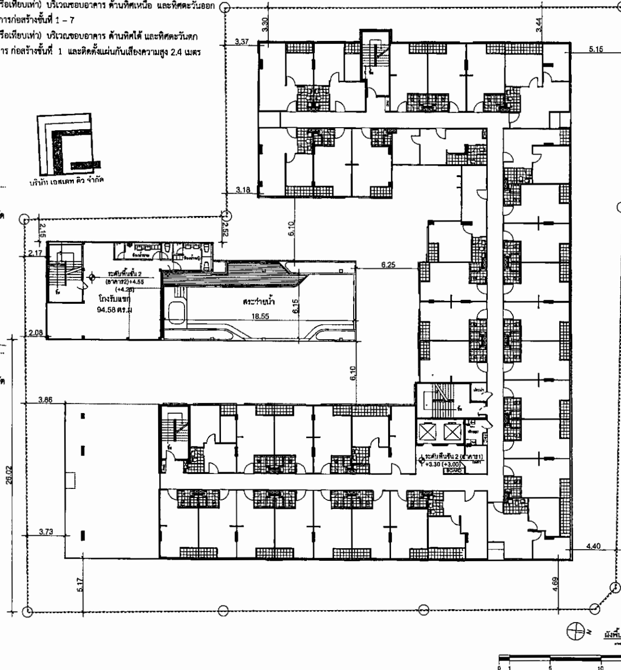
รูปที่ 4 แบบแสดงตำแหน่งแนวติดตั้งผนังกันเสียงในช่วงชั้นโครงสร้างอาคาร
