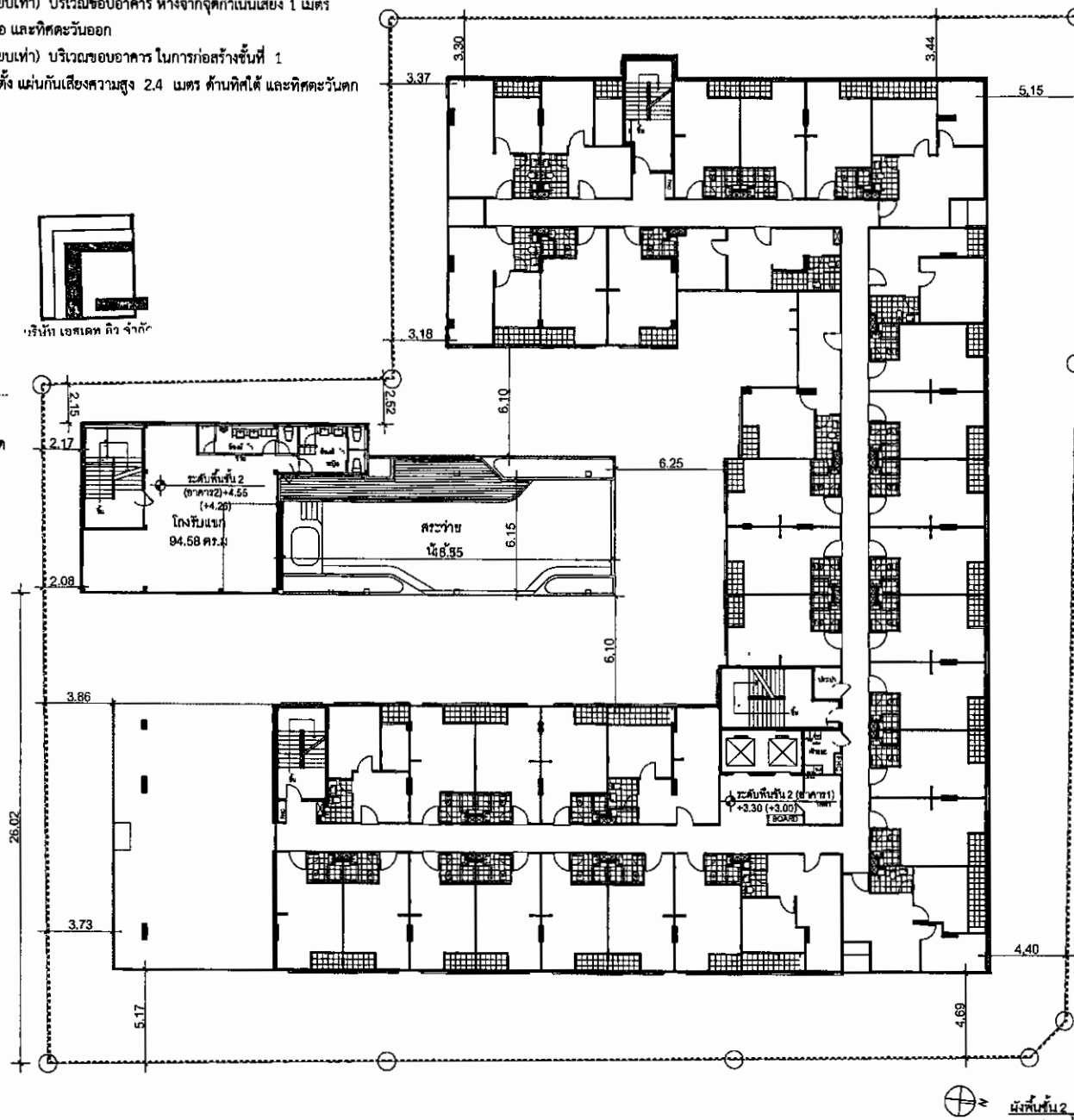
รูปที่ 5 แบบแสดงตำแหน่งแนวติดตั้งผนังกันเสียงในช่วงงานระบบสาธารณูปโภค ตกแต่งภายในและภายนอก
