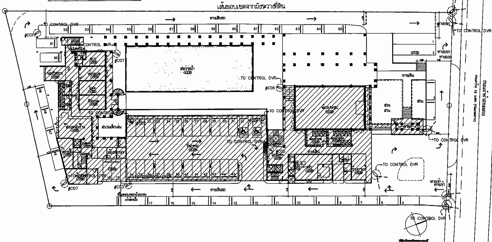
รูปที่ 13 ผังตำแหน่งกล้องวงจรปิด
