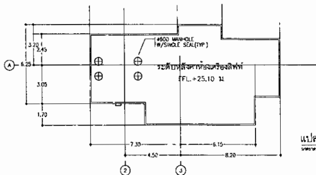
รูปที่ 4 (ต่อ) ตำแหน่งถังเก็บน้ำชั้นหลังคา
