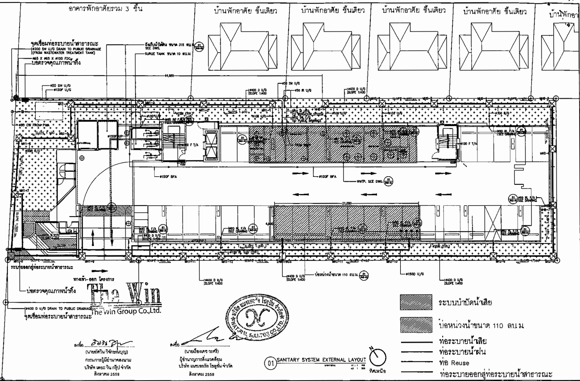
รูปที่ 6 ผังระบบระบายน้ำ
