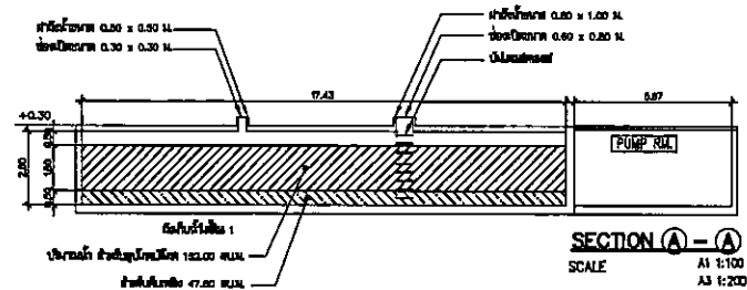
รูปที่ 8 แบบขยายถังเก็บน้ำฝนใต้ดิน
