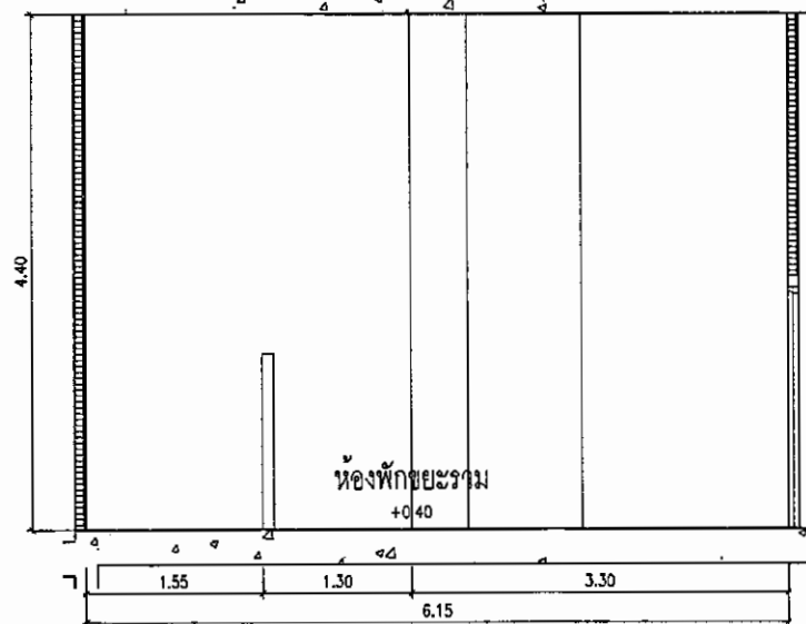
แปลนห้องพักรวมโครงการ SCALE 1:50
