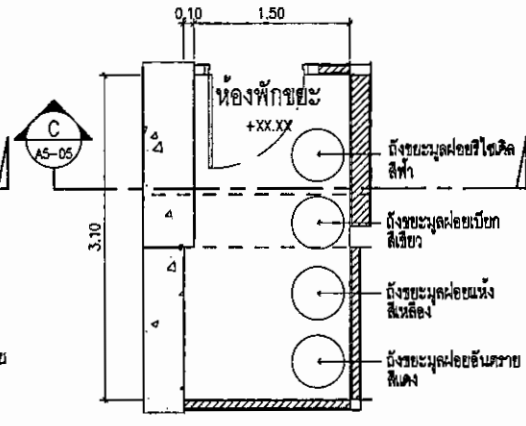
แปลนห้องพักรวม ชั้น 26 SCALE 1:50
