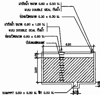
SECTION A - A SCALE A1 1:75 A3 1:150
