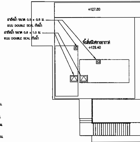
ผัดถังเก็บน้ำบาดาล SCALE A1 1:75 A3 1:150
