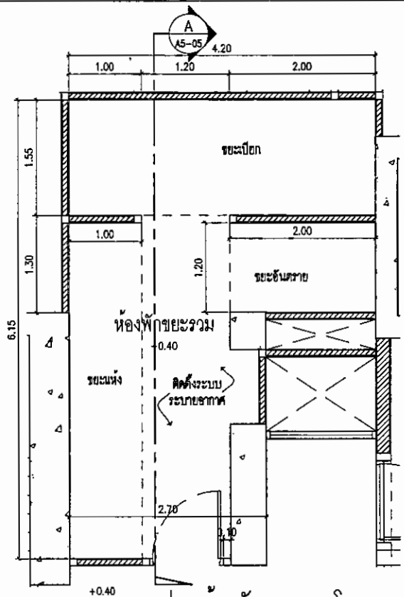
แปลนห้องพักรวมโครงการ SCALE 1:50
