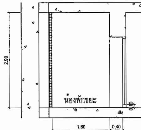
รูปตัด B SCALE 1:50
