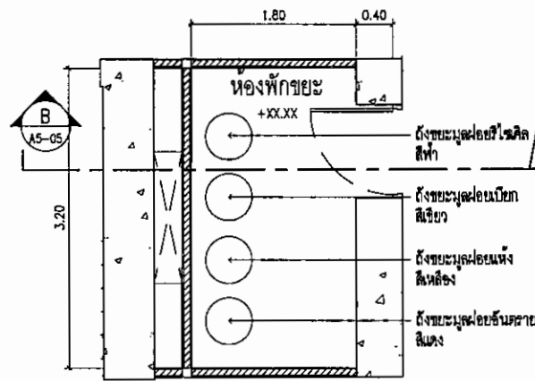
แปลนห้องพักรวม ชั้น 2-25, 27-38 SCALE 1:50
