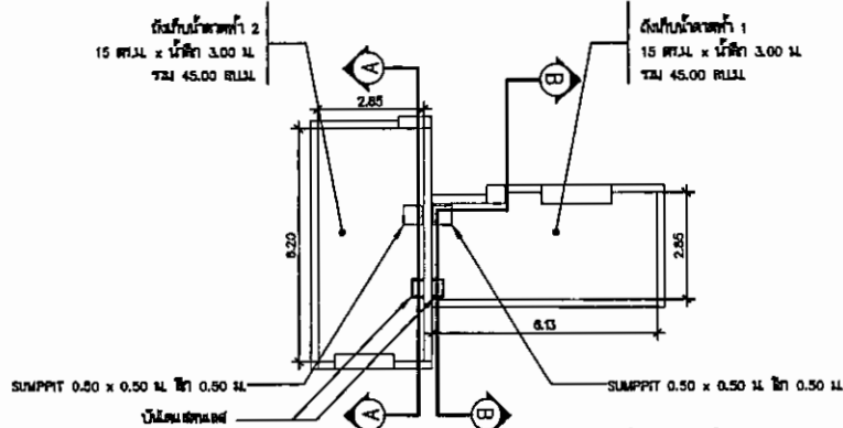
ถังเก็บน้ำบาดาล SCALE A1 1:75 A3 1:150
