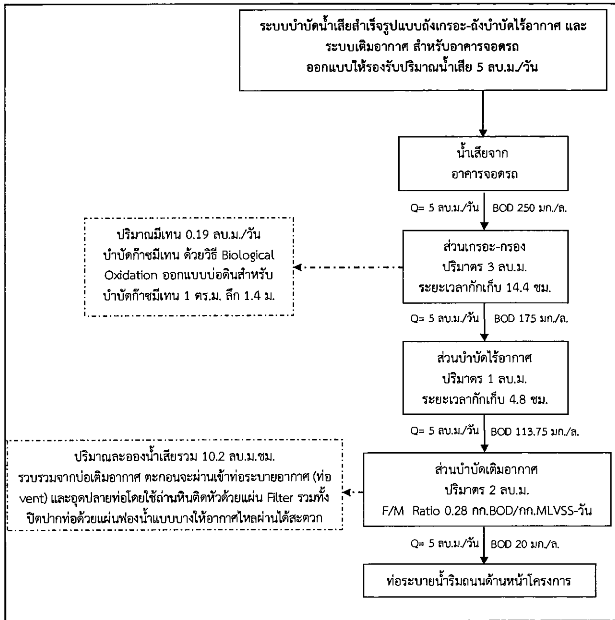
รูปที่ 4 แผนผังขั้นตอนการบำบัดน้ำเสียและสิ่งปฏิกูลสำเร็จรูปแบบถังเกรอะ-ถังบำบัดไร้อากาศ และระบบเติมอากาศ สำหรับอาคารจอดรถ
