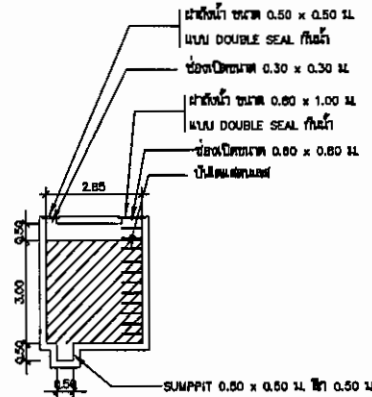
SECTION B - B SCALE A1 1:75 A3 1:150
