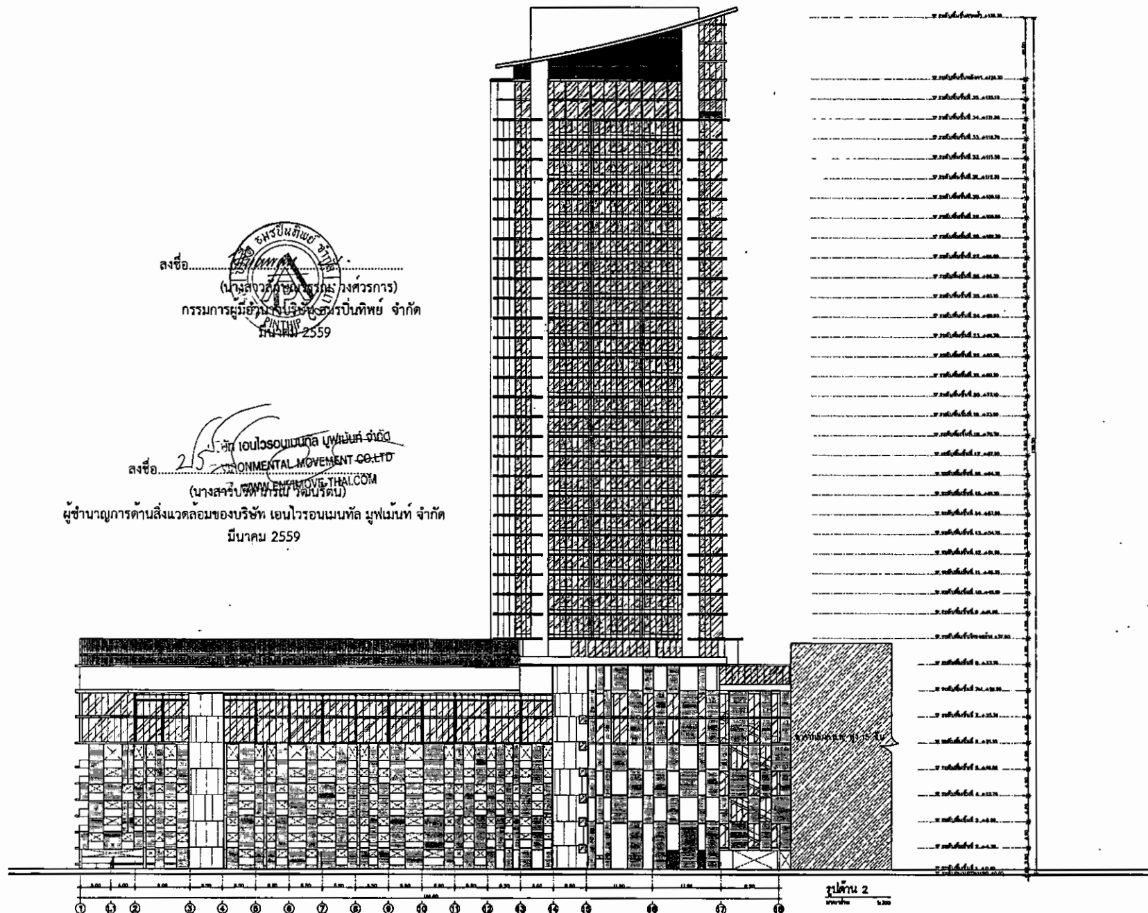
รูปที่ 18 รูปด้าน 2 ของทาวเวอร์ขนาดความสูง 35 ชั้น
