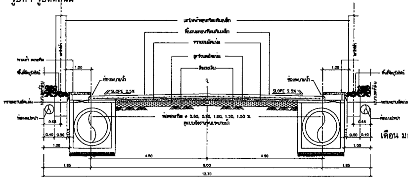
แบบขยายหน้าตัดถนนกว้าง 12.70 ม. มาตรา 1:50
