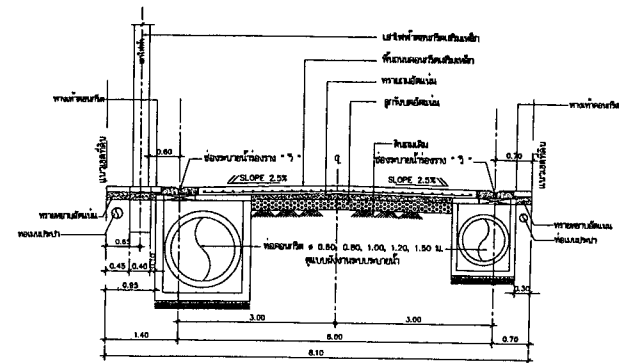
แบบขยายหน้าตัดถนนกว้าง 8.10 ม. มาตรา 1:50
