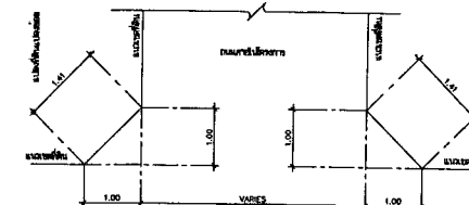
แบบขยายการระบายน้ำ มาตรา 1:50
