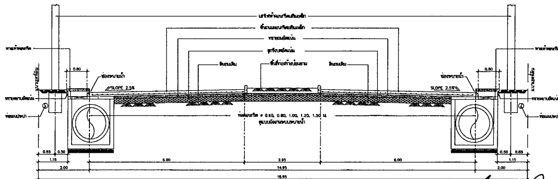
แบบขยายหน้าตัดถนนกว้าง 18.95 ม. มาตรา 1:50
