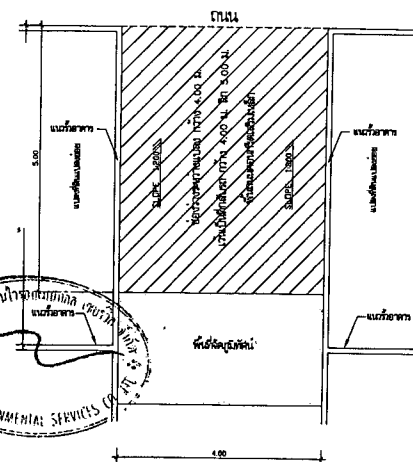
แบบขยายช่องว่างระหว่างแปลงกว้าง 4.00 ม. มาตรา 1:50
