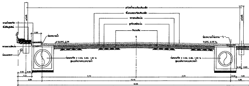
แบบขยายหน้าตัดถนนกว้าง 18.95 ม. ของบริษัทก่อสร้างจำกัด โฉมเลขที่ 6672 มาตรา 1:50
