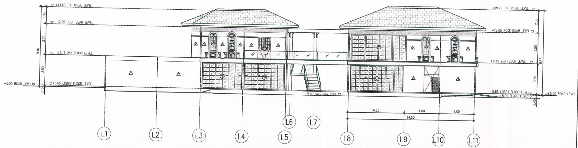
ELEVATION.1 SCALE 1 : 200
