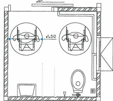
แบบขยายห้องน้ำผู้พิการ
