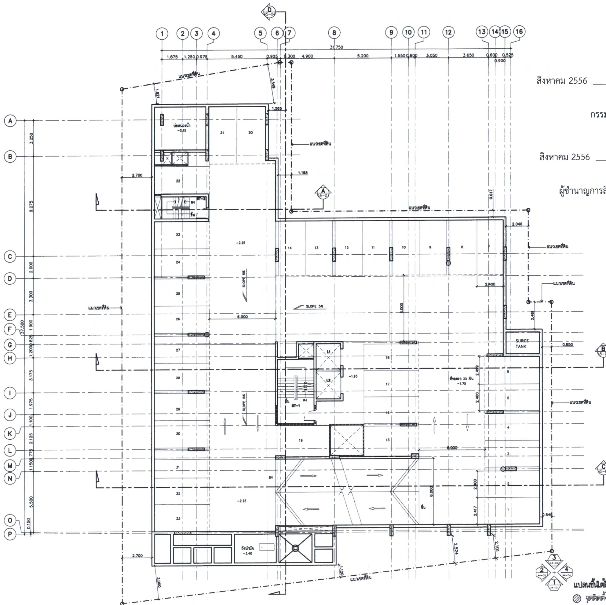
รูปที่ 4 ผังแสดงพื้นที่จอดรถของโครงการชั้นใต้ดิน 1
