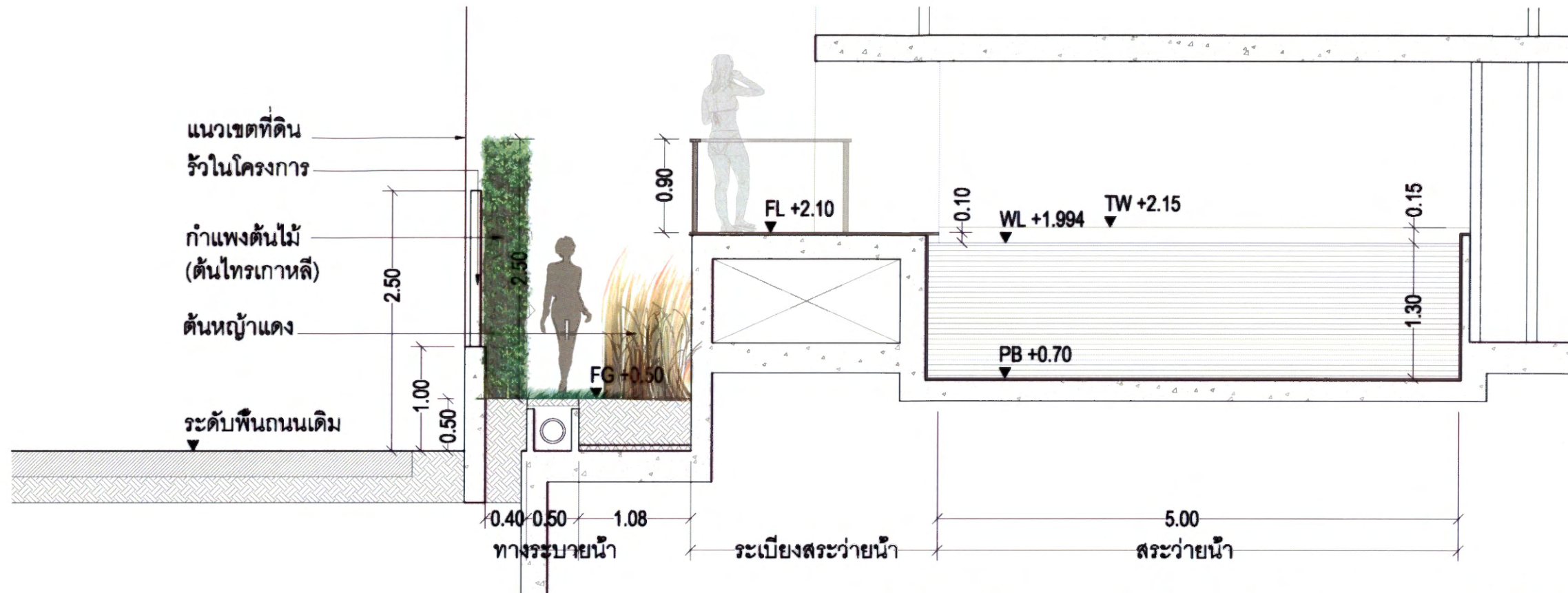
A รูปตัด A สระว่ายน้ำ ทางเดินรอบโครงการและแนวต้นไม้
