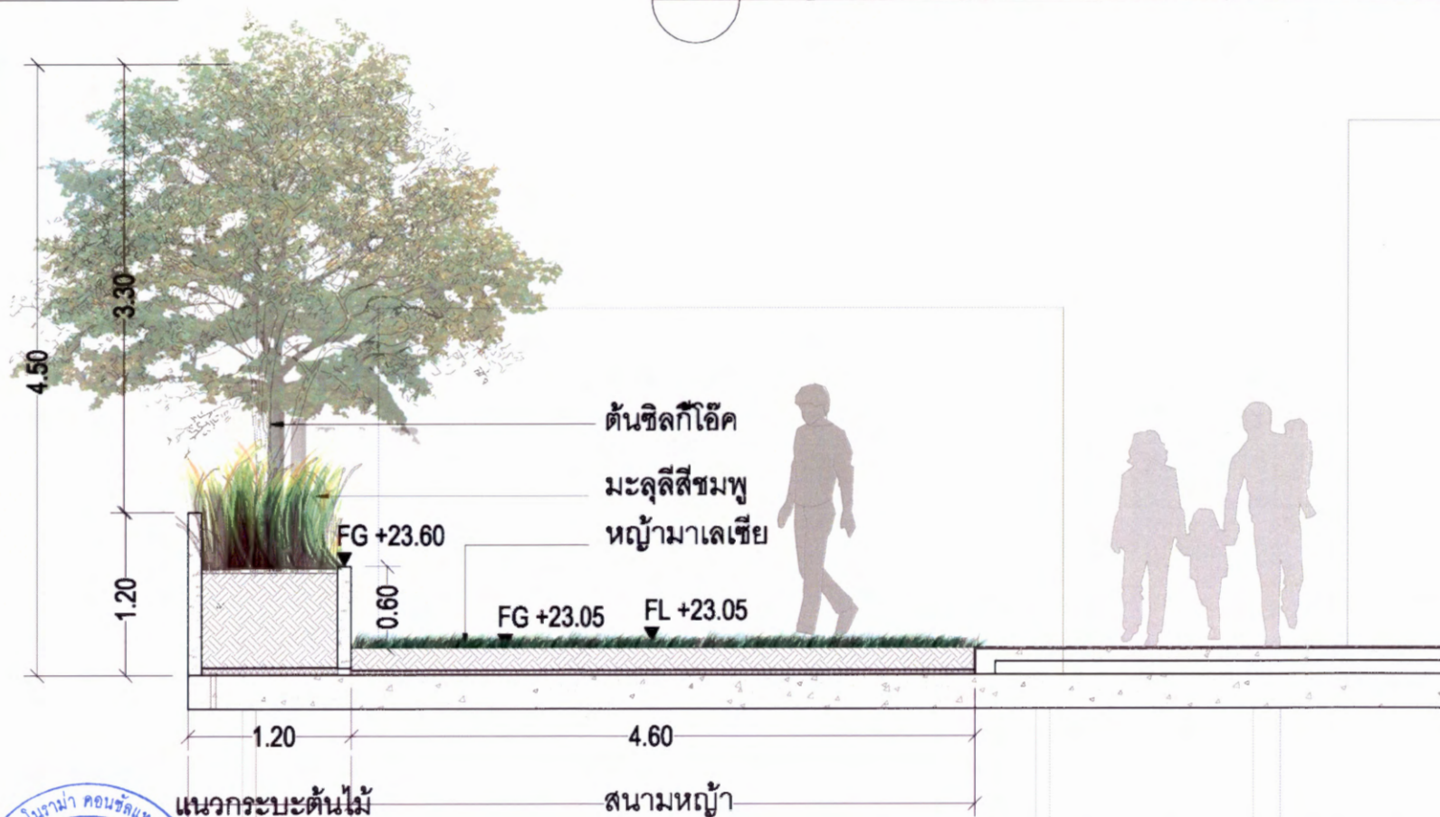
D รูปตัด D ห้องขยะและพื้นที่ปลูกต้นไม้ด้านข้าง
