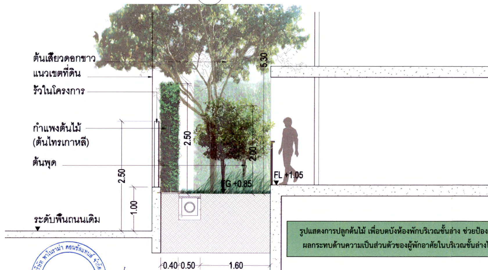
B รูปตัด B ที่ระบียงชั้น1 และแนวต้นไม้หน้าห้อง
