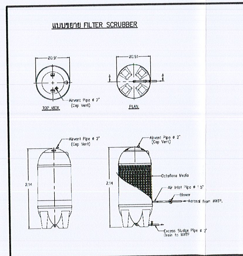
รูปที่ 11 แบบขยายและรูปตัดบ่อปรับสภาพน้ำเสียตอนปลาย แบบแปลนและรูปตัดบ่อกำจัดก๊าซมีเทน และแบบขยายท่อบายอากาศที่ติดตั้ง Filter เพื่อจำกัด Aerosol
