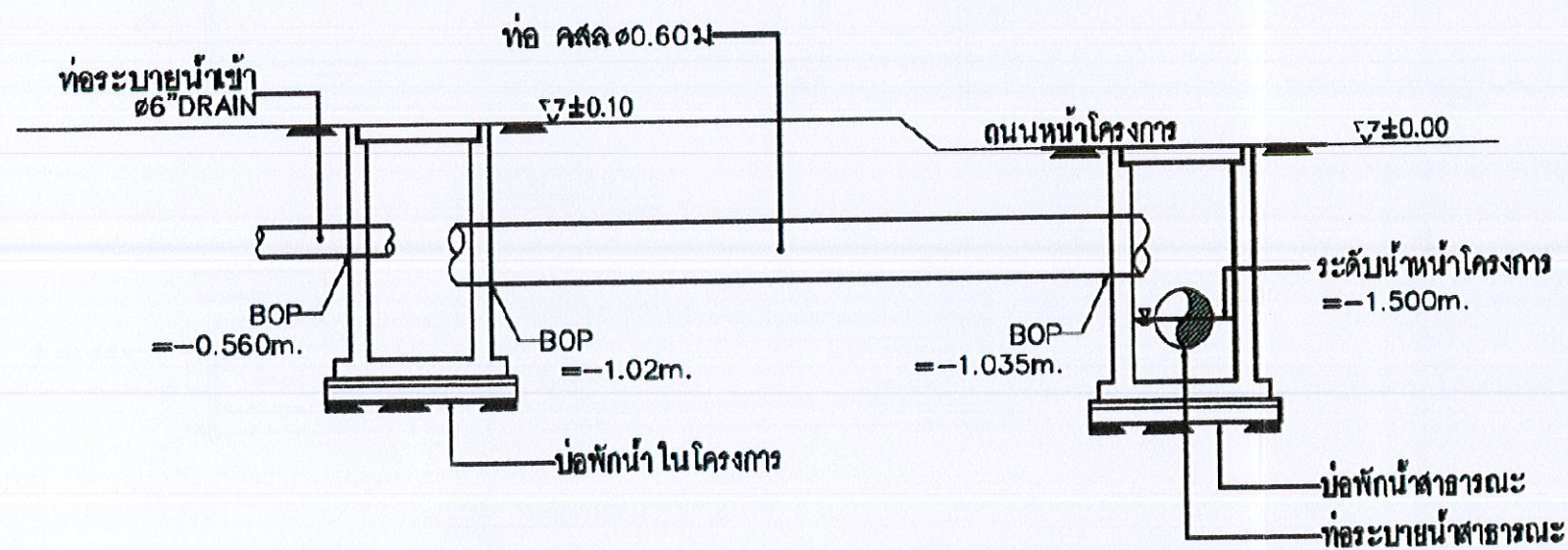
แบบขยายจุดเชื่อมต่อท่อระบายน้ำของโครงการกับบ่อพักน้ำสาธารณะ 2 ในชั้นวางดิน
