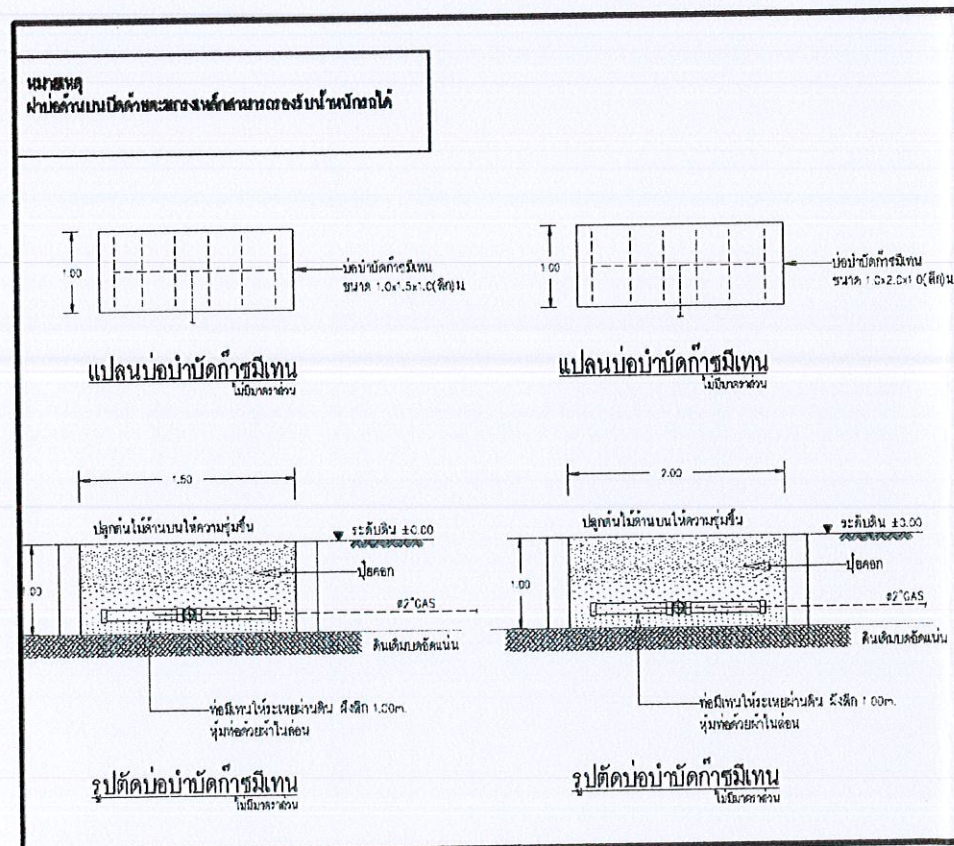
รูปที่ 11 แบบขยายและรูปตัดบ่อปรับสภาพน้ำเสียตอนปลาย แบบแปลนและรูปตัดบ่อกำจัดก๊าซมีเทน และแบบขยายท่อบายอากาศที่ติดตั้ง Filter เพื่อจำกัด Aerosol
