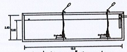
รูปตัดบ่อรับสภาพน้ำเสียตอนปลาย
