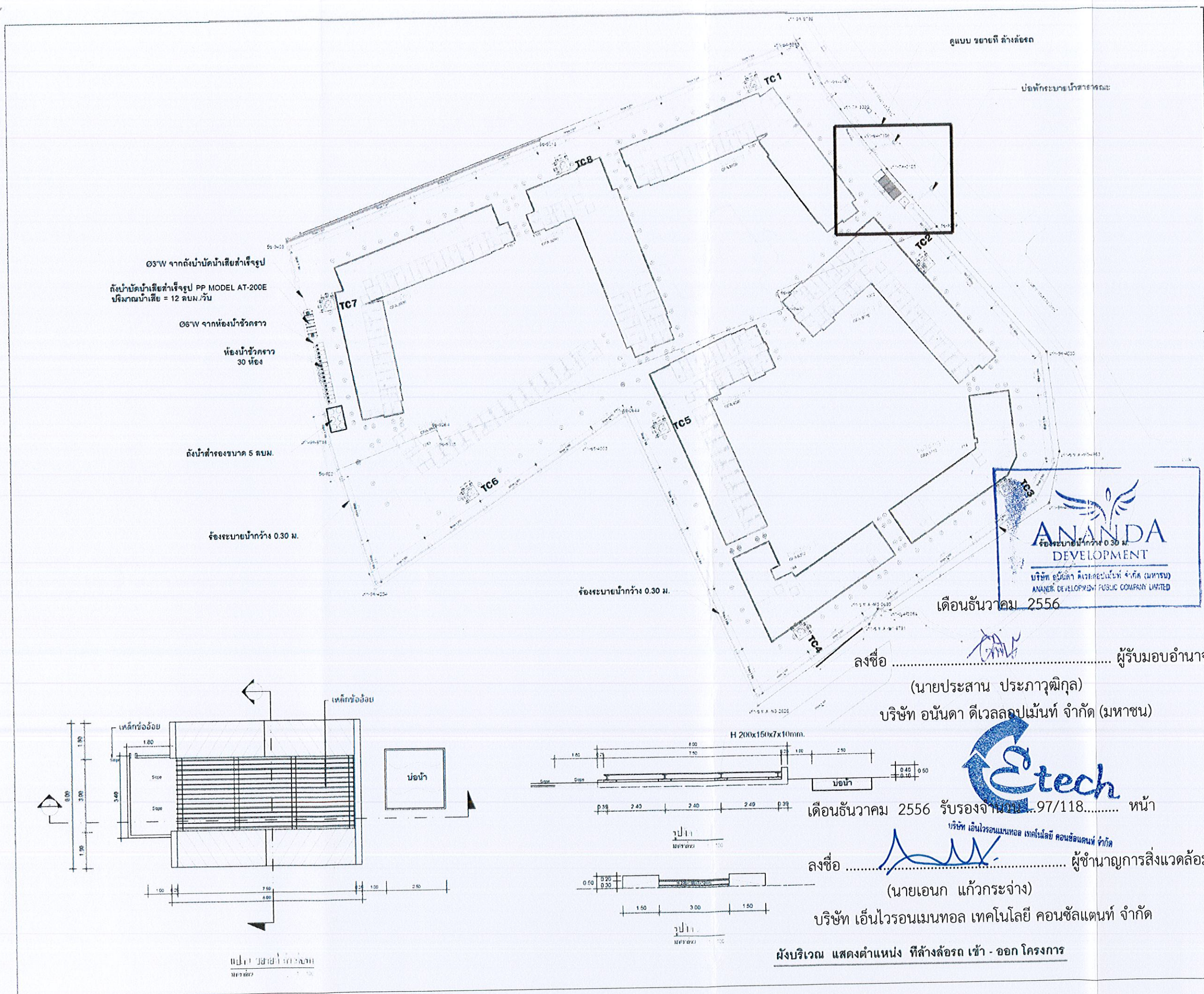
รูปที่ 5 ผังระบบสุขาภิบาลในพื้นที่ก่อสร้าง และแบบขยายบริเวณล้างลอร์ดในบริเวณพื้นที่ก่อสร้างโครงการ
