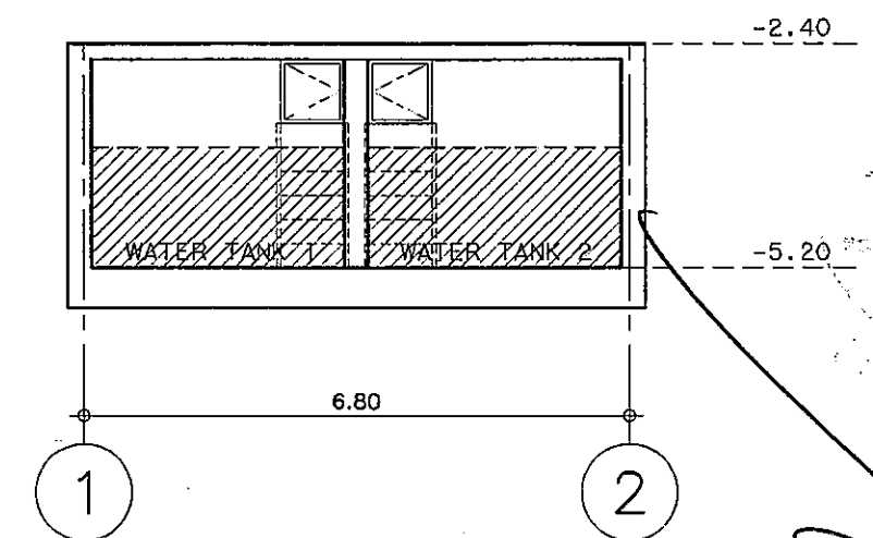
SECTION 2 SCALE 1 : 50
