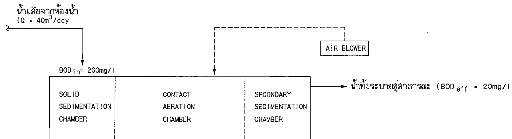
DIAGRAM ระบบบำบัดน้ำเสีย
