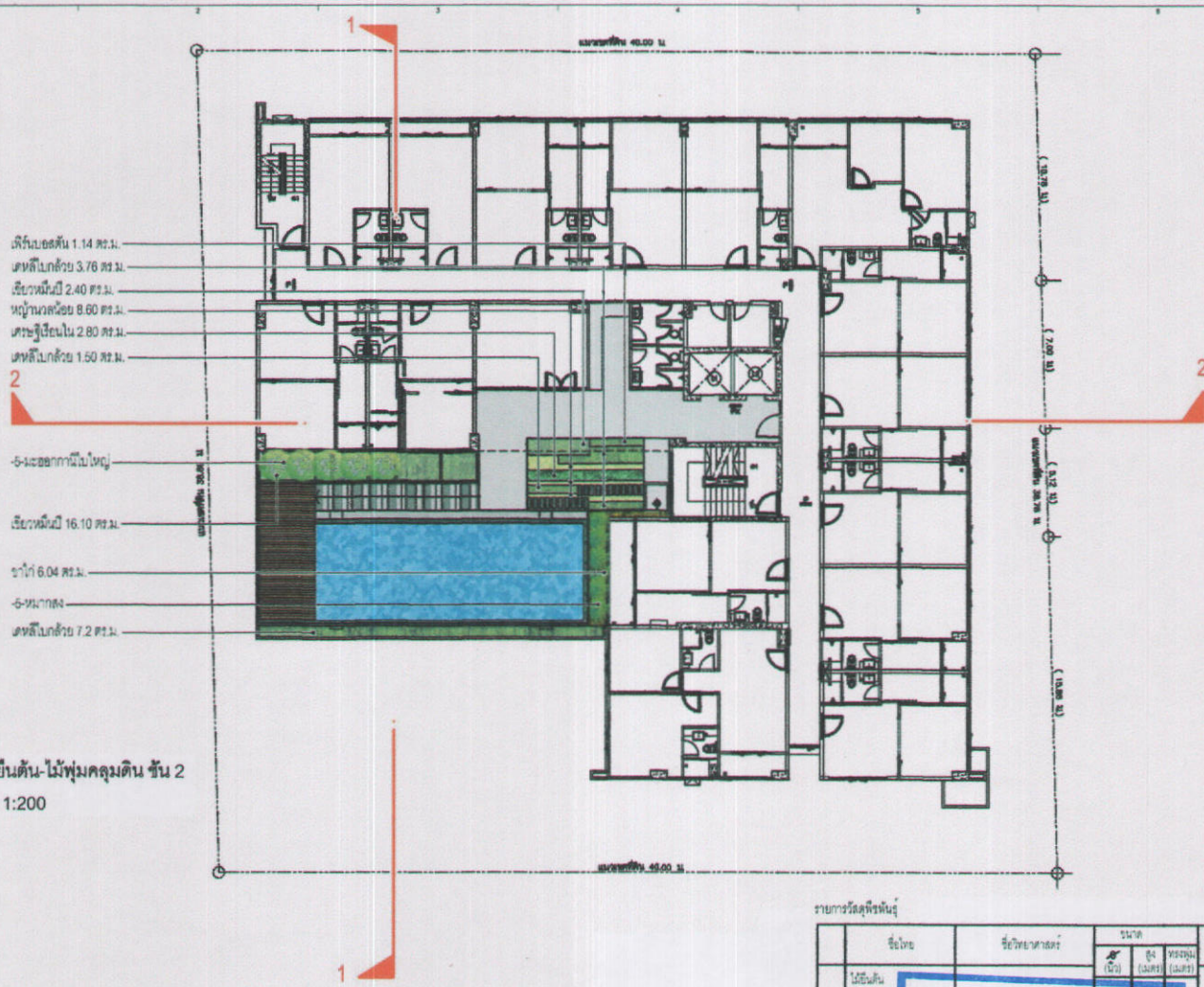
รูปที่ 12 (ต่อ) ผังแสดงพื้นที่สีเขียวของโครงการ
