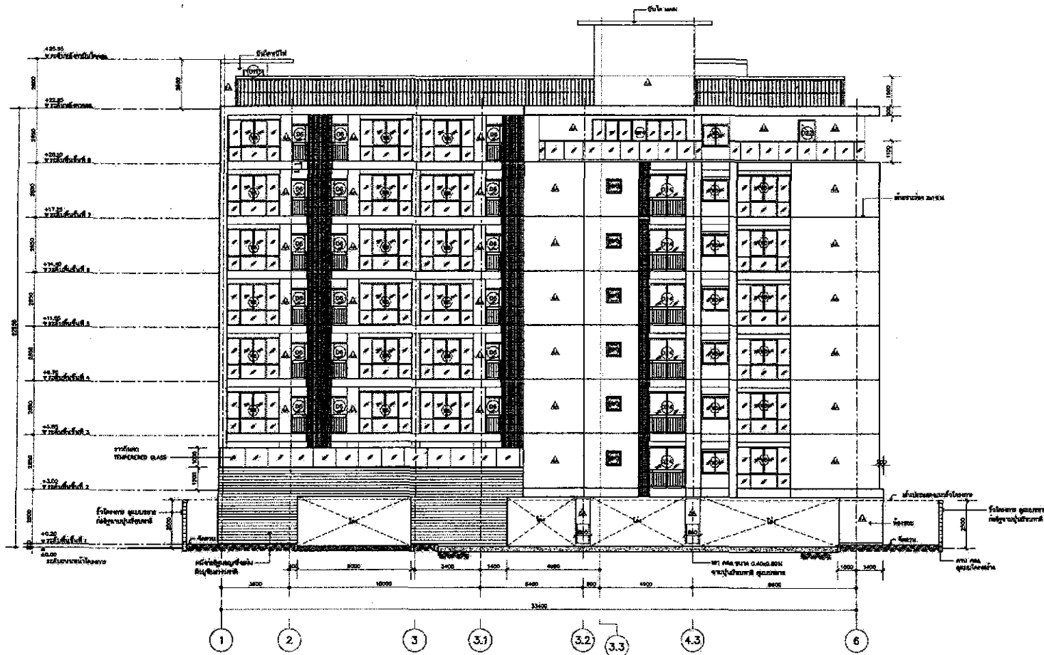
รูปที่ 4 รูปด้านของโครงการ
