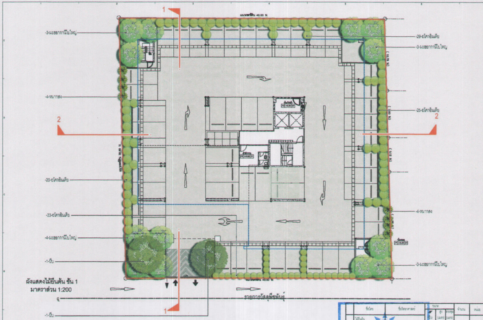
รูปที่ 12 ผังแสดงพื้นที่สีเขียวของโครงการ
