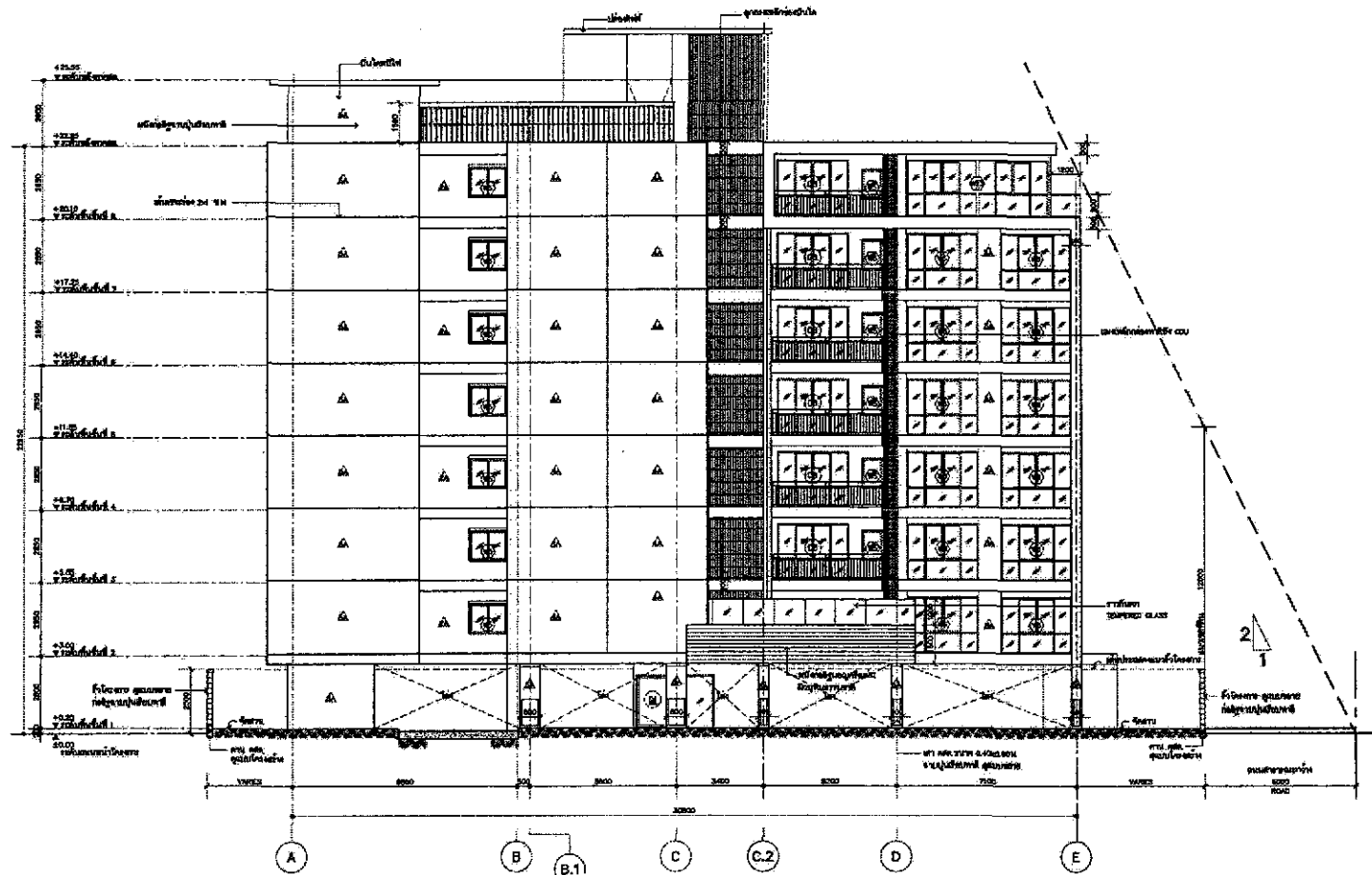
รูปที่ 4 (ต่อ) รูปด้านของโครงการ
