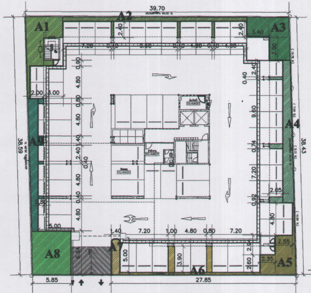
ผังแสดงพื้นที่สีเขียว-ชั้น 1
