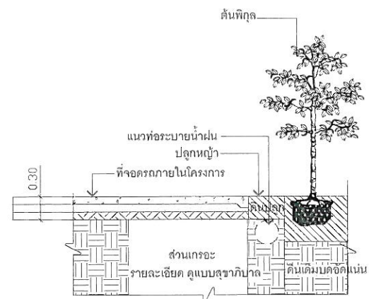
รูปตัด 2 แสดงการปลูกไม้ต้นและไม้คลุมดิน เหนือบ่อบำบัด
